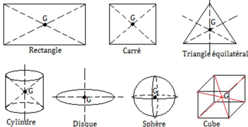
Figure 7.4 : Centre d'inertie de quelques solides particuliers.
