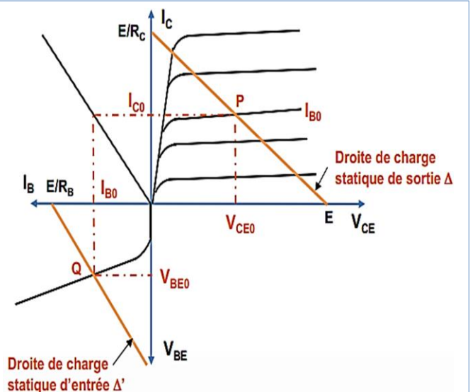
Polarisation du transistor : Point de fonctionnement.
