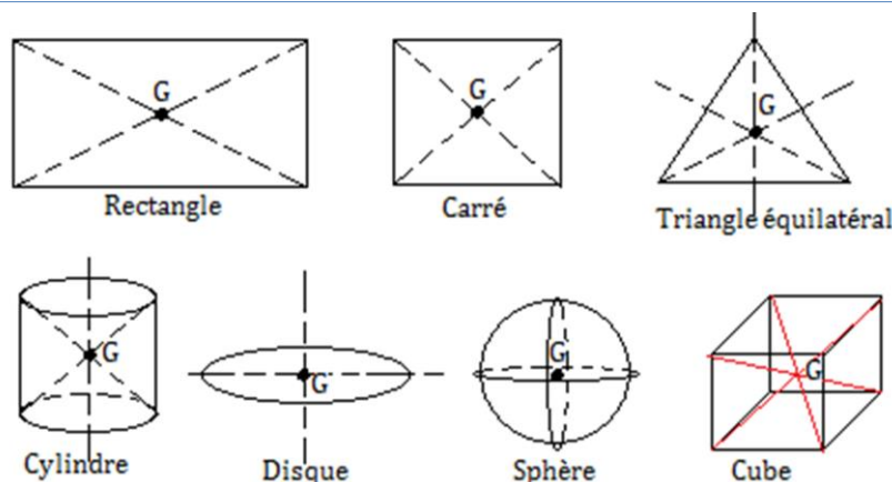
Figure 7.4 : Centre d'inertie de quelques solides particuliers.
