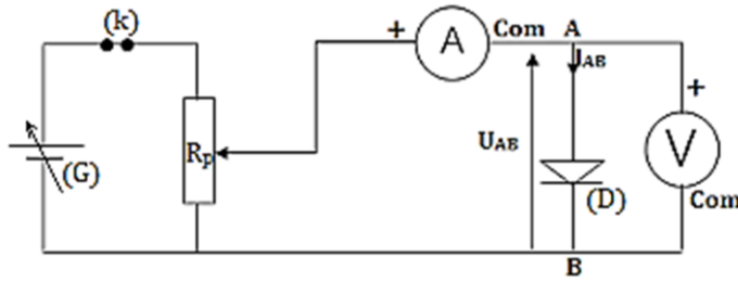
Figure 13.8 : Dispositif expérimental
