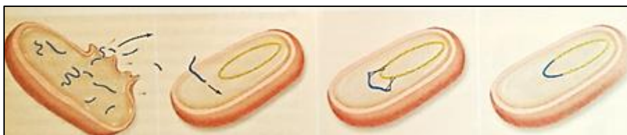
Figure 75 : Transformation bactérienne
