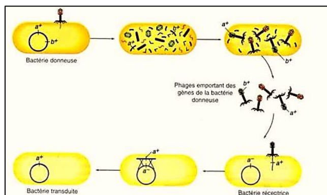
Figure 74 : Transduction bactérienne
