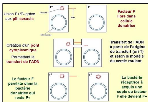
Figure 73 : Conjugaison bactérienne
