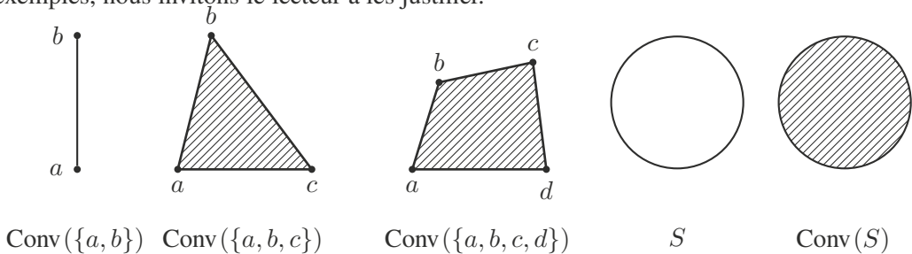
FIGURE II.1.3 – Exemples d'enveloppes convexes.
