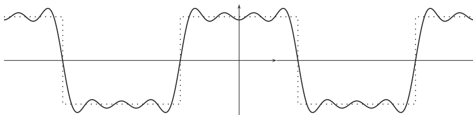
FIGURE II.4.1 – La somme des quatre premiers termes de la série \sum_{n \geq 0} \frac{1}{2n+1} \cos(2n+1)x (en trait continu) et de la fonction 2\pi -périodique qui vaut \pi/4 pour |x| < \pi/2 et -\pi/4 pour \pi/2 < |x| < \pi (en pointillés).
