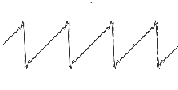
FIGURE II.4.4 – La somme partielle S_{10}(f) d'une fonction en dents de scie.
