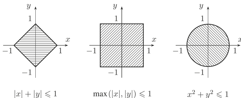
FIGURE II.1.1 – La boule unité dépend de la norme choisie.
