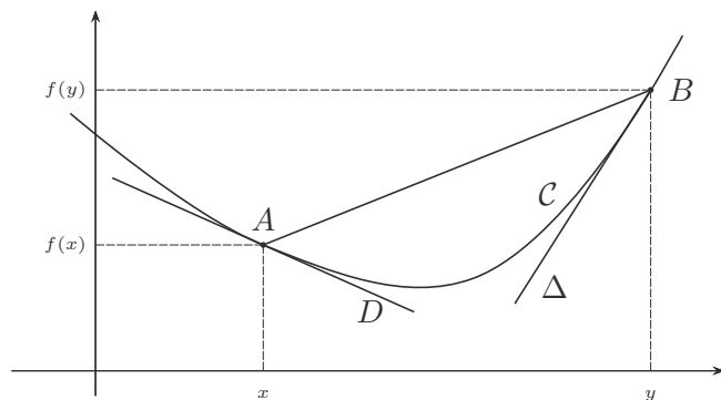
FIGURE II.1.5 – La courbe est au-dessus de chacune de ses tangentes.
