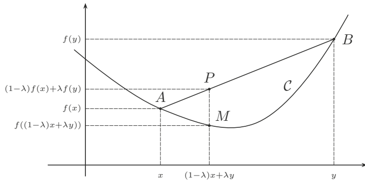
FIGURE II.1.4 – La courbe est au-dessous de ses cordes : f est convexe.
