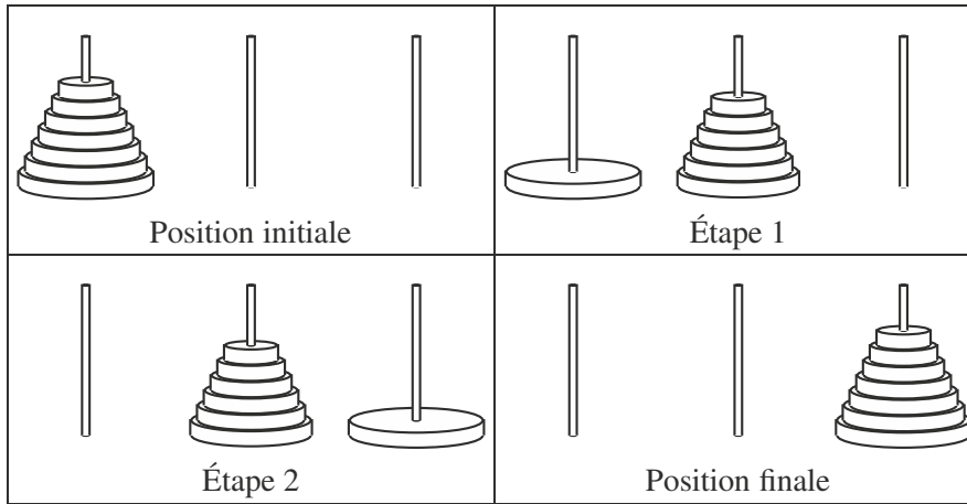
FIGURE I.8.1 – Le problème des tours de Hanoi
