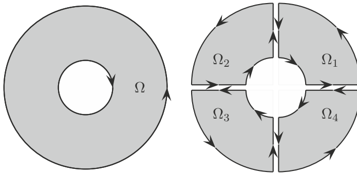
FIGURE II.5.1 – Découpage d'une couronne en quatre morceaux horizontalement et verticalement simples
