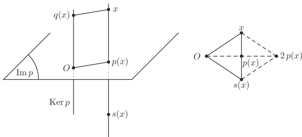
FIGURE I.4.2 – Projection et symétrie orthogonale : x + s(x) = 2p(x) et x = q(x) + p(x) .
