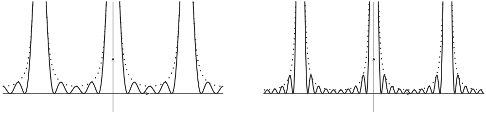
FIGURE II.4.3 – Les noyaux de Féjer pour N = 5 et N = 10 .
