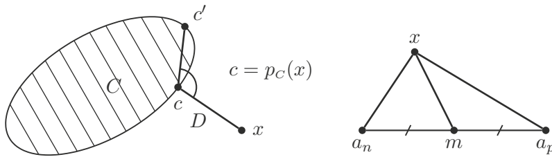
FIGURE II.1.6 – Projection sur un convexe complet.
