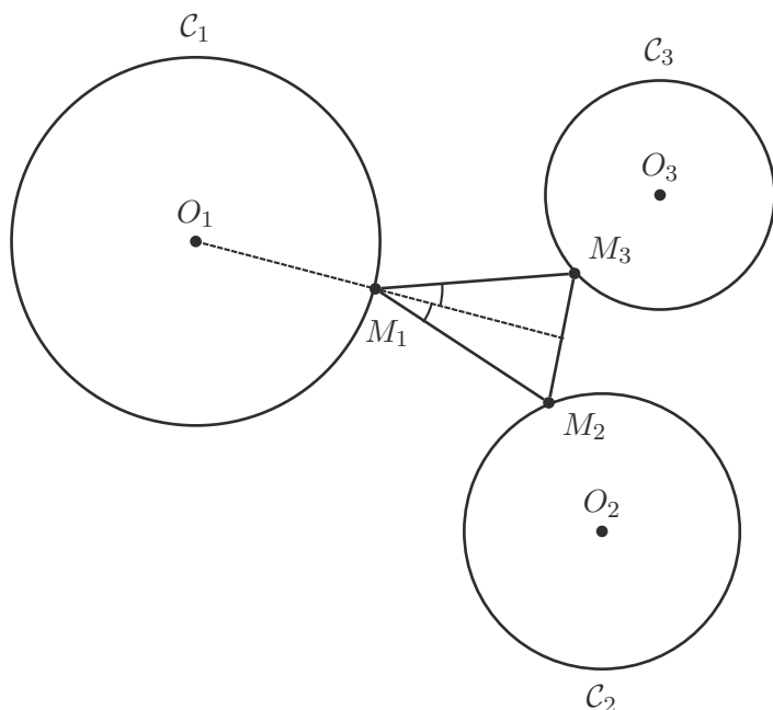
FIGURE II.1.2 – Triangle de périmètre minimum.
