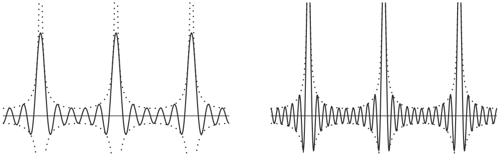
FIGURE II.4.2 – Les noyaux de Dirichlet pour N = 5 et N = 10 .
