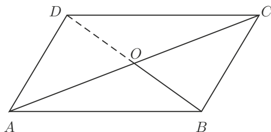
FIGURE I.4.1 – Formule de la médiane.
