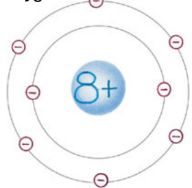
oxygène
