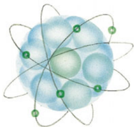
azote
