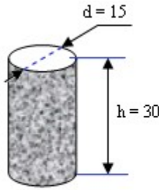
La dimension de l'éprouvette pour mesurer la résistance en compression
