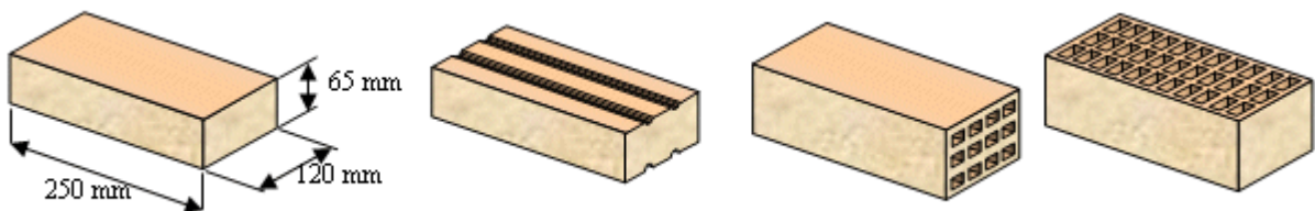
fig. 7.1: Briques pleines et perforées
