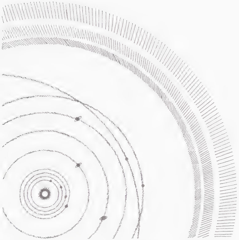
*Figure 8. Le système solaire.
