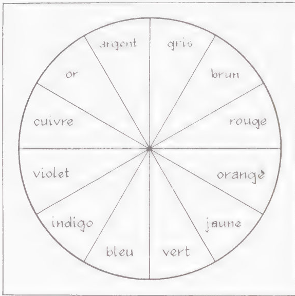
*Figure 11. Le spectre terrestre.
