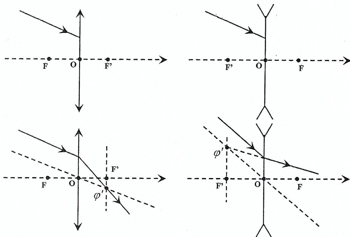
Figure 11 : Tracé d'un rayon émergent
