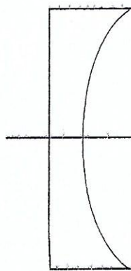
Lentille plan-concave
