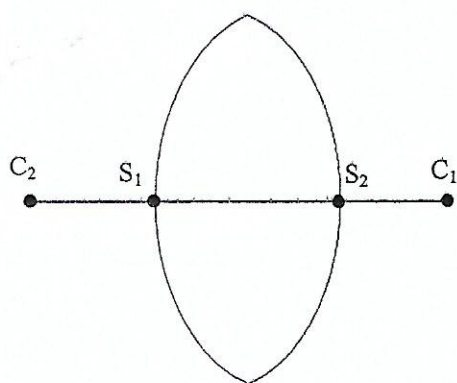
Lentille biconvexe
