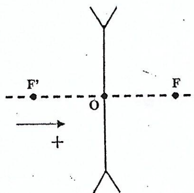
Figure 7 : Lentille divergente
