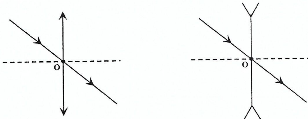
Figure 8 : Rayon passant par le centre optique
