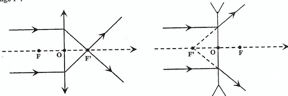
Figure 9 : Rayons incidents parallèles à l'axe optique
