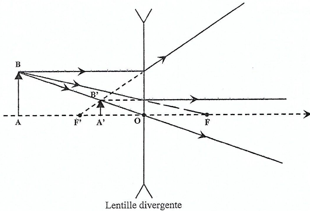
Figure 13 : Construction d'image à travers une lentille mince
