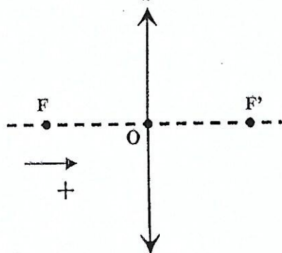
Figure 6 : Lentille convergente
