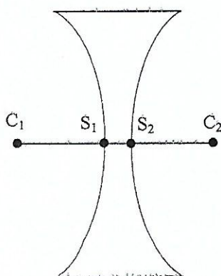
Lentille biconcave
