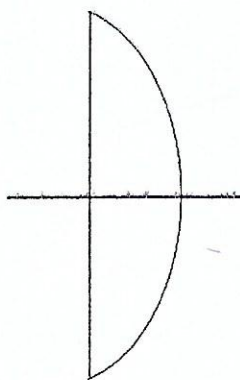
Lentille plan-convexe
