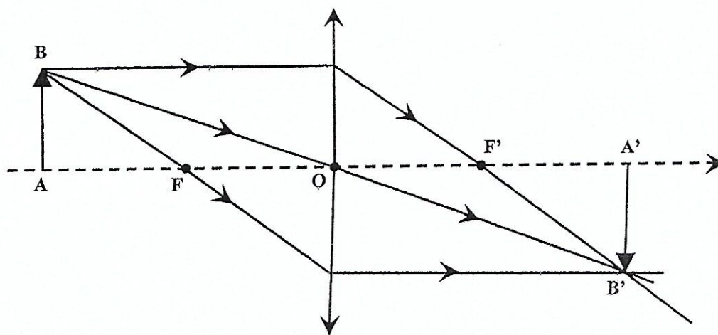
Lentille convergente
