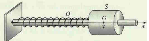
Doc. 7 Oscillateur élastique horizontal en translation. O coïncide avec la position G_0 de G lorsque le ressort a sa longueur naturelle (équilibre du système {solide-ressort}).
