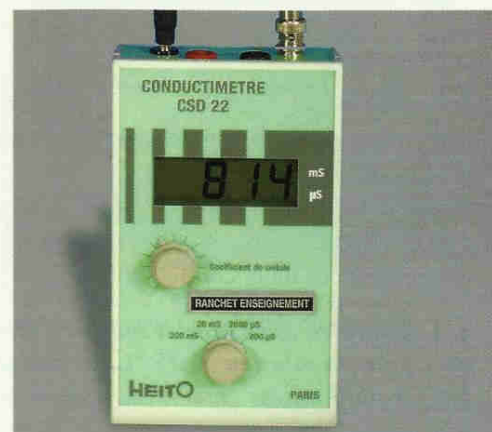
Doc. 7 Un conductimètre relié à une cellule conductimétrique permet de connaître la conductivité de la solution.
