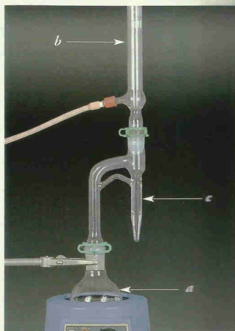
Doc. 12 Appareil de DEAN et STARK.
