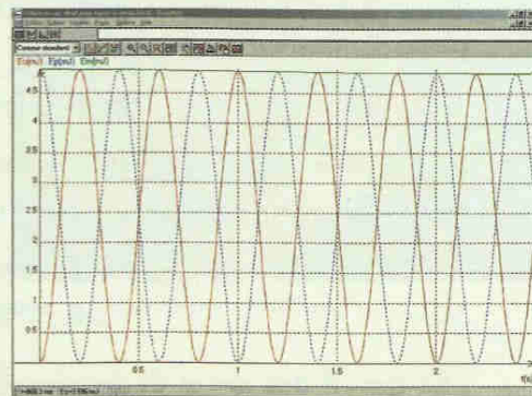
Doc. 9 Représentation des énergies cinétique et potentielle élastique en fonction du temps : quand une énergie est maximale, l'autre est nulle. E_C est représentée en rouge, E_{P\text{ élas}} en bleu et E_M en vert.
