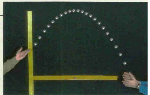
Doc. 13 Mouvement d'une bille enregistré au caméscope.
