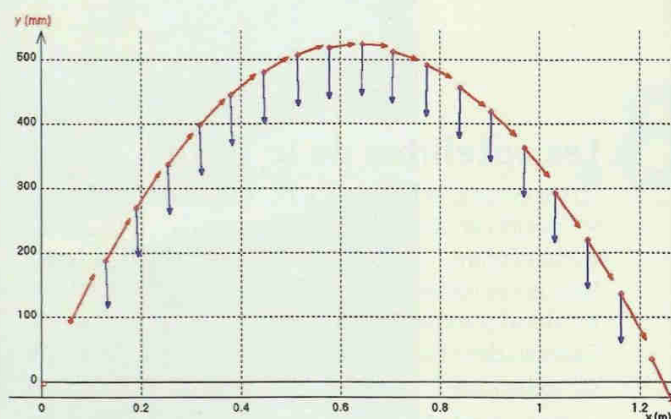
Doc. 2 Vecteurs vitesse (en rouge) et accélération (en bleu) au cours du mouvement.
