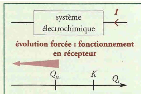
Doc. 4 Transformation forcée d'un système électrochimique.
