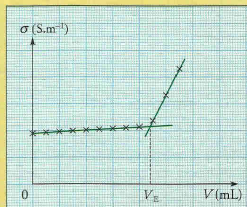
Doc. 3 Changement de pente à l'équivalence.
