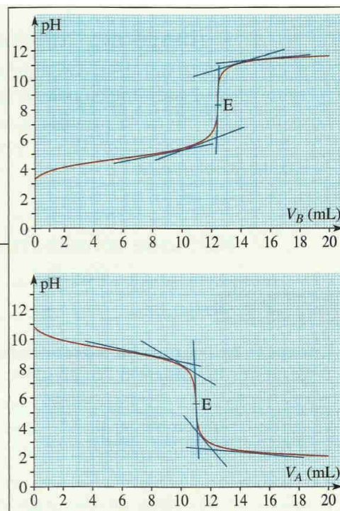
Doc. 8 Tracé des tangentes aux graphes (a) pour le graphe pH = f(V_B) (b) pour le graphe pH = f(V_A) .
