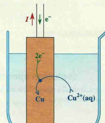
Doc. 11 Réduction des ions cuivre (II) \text{Cu}^{2+} à l'électrode de cuivre. Le gain d'électrons s'effectue à la surface de l'électrode.
