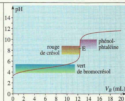
Doc. 11 Courbe \text{pH} = f(V_B) et zone de virage d'indicateurs colorés.
