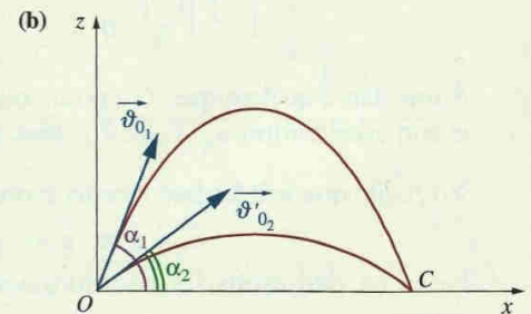
Doc. 5 Trajectoires d'un projectile.
