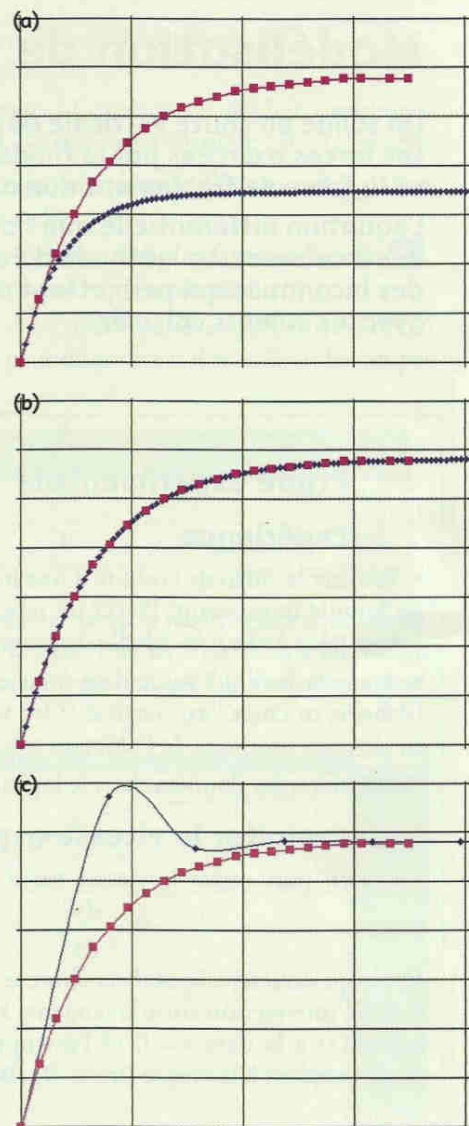
Doc. 18 On cherche à superposer la courbe obtenue par la méthode d'EULER (en bleu) avec la courbe expérimentale (en rose).
