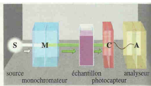
Doc. 13 Schéma de principe d'un spectrophotomètre.
