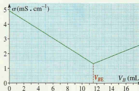
Doc. 7 Suivi conductimétrique d'un titrage acido-basique.
