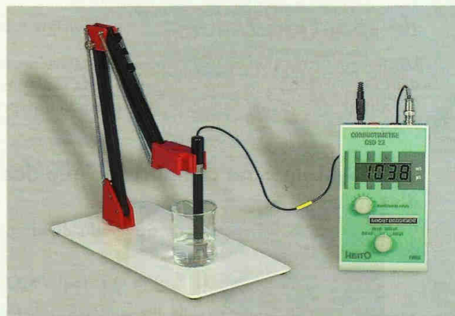
Doc. 1 Mesure de la conductivité : \sigma = 1\,038 \text{ } \mu\text{S} \cdot \text{cm}^{-1} .
