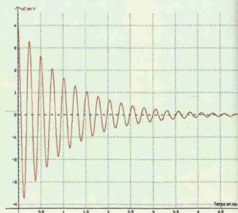
Doc. 2 Oscillations électriques libres amorties.
