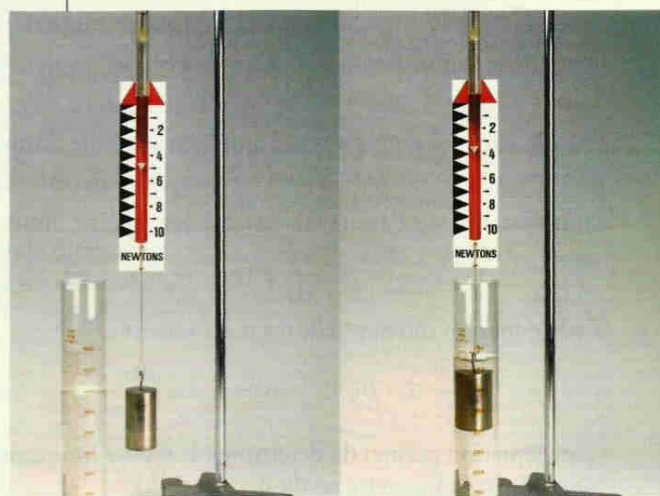
Doc. 13 Étude expérimentale de la poussée d'ARCHIMÈDE.
