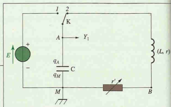
Doc. 1 Montage expérimental permettant d'étudier un circuit (R, L, C) série.
