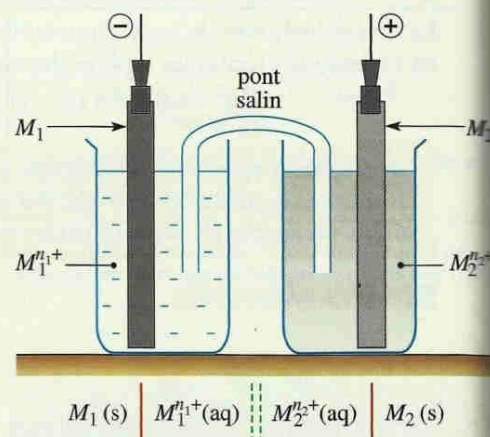
Doc. 8 Constitution d'une pile.
