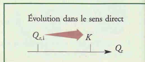
Doc. 13 Le critère d'évolution spontanée permet de prévoir le fonctionnement de la pile.
