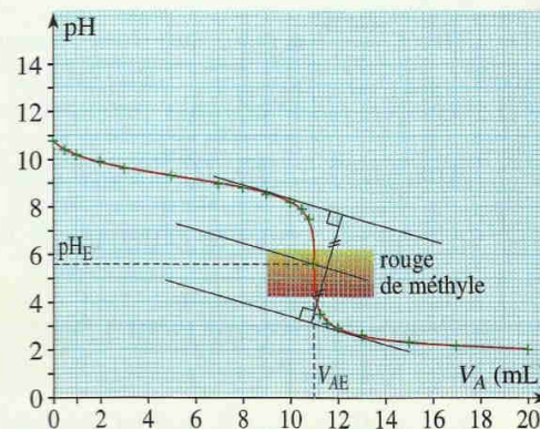
Doc. 12 Choix d'un indicateur coloré adapté.
