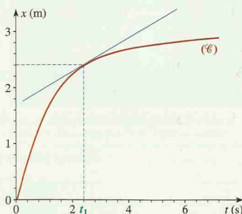
Doc. 6 La tangente à la courbe x(t) , pour la date t_1 , permet de déterminer la vitesse du mobile P à cet instant.
