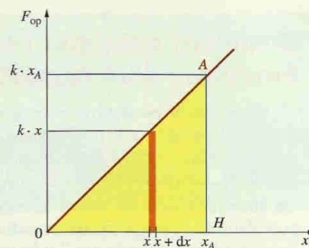
Doc. 5 Intégration graphique. La droite OA a pour équation F_{\text{op}} = k \cdot x .
