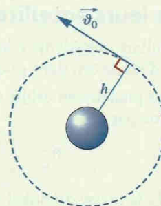
Doc. 14 Pour une satellisation circulaire à une altitude h donnée, la vitesse de lancement \vec{\vartheta}_0 est imposée.
