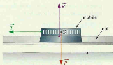
Doc. 6 Bilan des forces extérieures s'exerçant sur le mobile.
