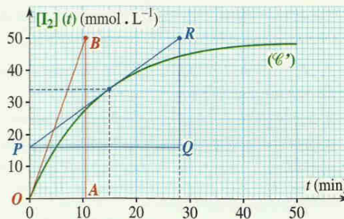
Doc. 8 Détermination des vitesses volumiques de réaction.
