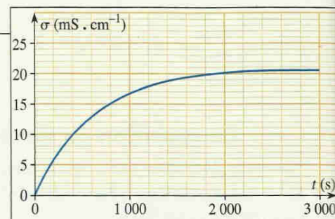
Doc. 9 Aspect de la courbe \sigma(t) .
