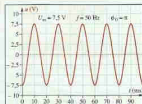
Doc. 5 Tension modélisée par la fonction mathématique : u(t) = 7,5 \cdot \cos(2\pi \cdot 50t + \pi) .
