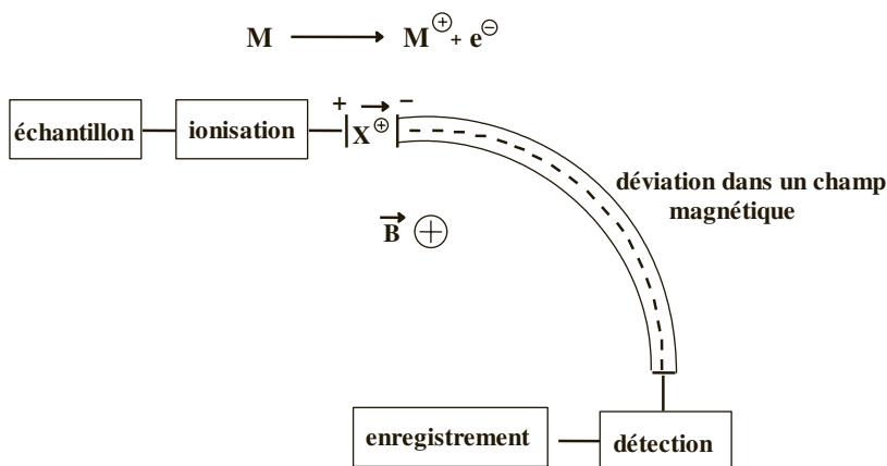
Figure 4.15 Principe du spectromètre de masse.
