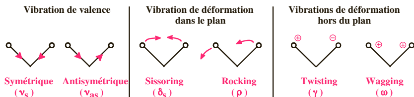
Figure 4.6 Différentes vibrations d'une molécule triatomique.
