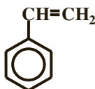
styrène (vinylbenzène)
