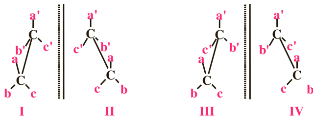
Figure 2.17 Stéréoisomères avec deux carbones asymétriques.
