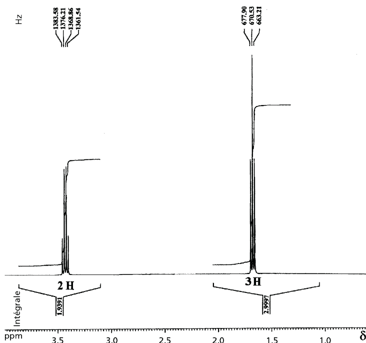
Figure 4.12 Spectre de RMN du bromoéthane ( \text{CH}_3\text{-CH}_2\text{-Br} ).
