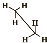
Conformation décalée
