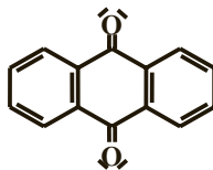
antraquinone
