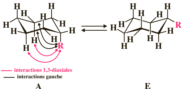
Figure 2.27 Équilibre chaïse ⇌ chaïse des cyclohexanes substitués.
