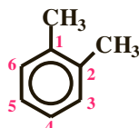
orthoxyène (1,2-diméthylbenzène)
