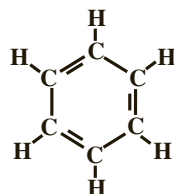
benzène
