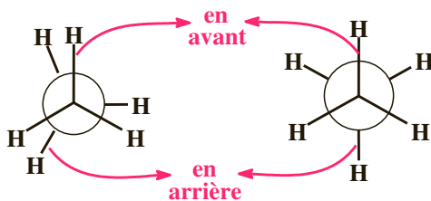
Conformation éclipsée
