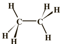
Conformation décalée
