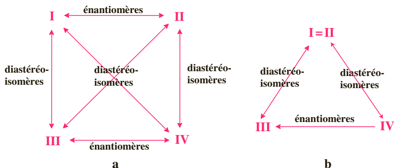
Figure 2.18 Différentes relations de stéréoisomérisation des composés I , II , III et IV . (a) Cas général. (b) Cas où les substituants liés aux carbones asymétriques sont deux à deux identiques ( a = a' , b = b' , c = c' ).
