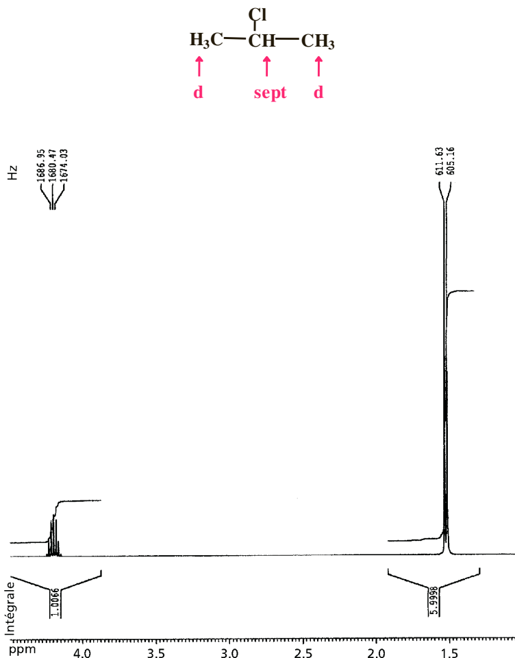
Figure 4.13 Spectre de RMN du 2-chloropropane ( \text{CH}_3\text{-CHCl-CH}_3 ).
