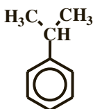
cumène (isopropylbenzène)
