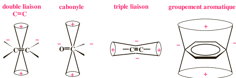
Figure 4.10 Cônes d'anisotropie de quelques nuages \pi .
