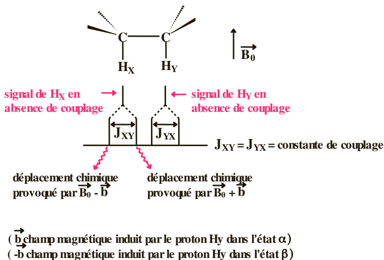
Figure 4.11 Schéma de principe du couplage spin-spin.
