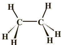
Conformation éclipsée
