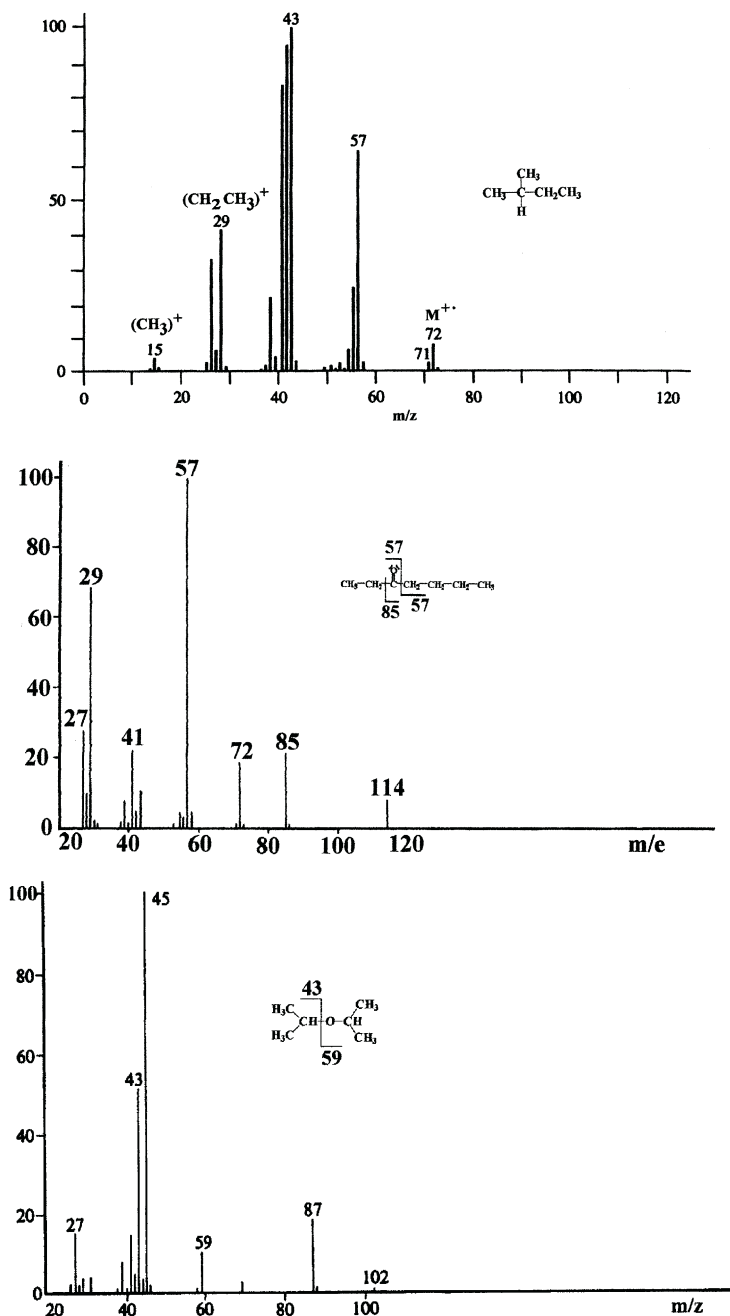
Figure 4.16 Exemples de spectres de masse.
