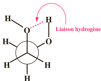
Figure 2.12 Forme gauche de l'éthane-1,2-diol (représentation de Newman).
