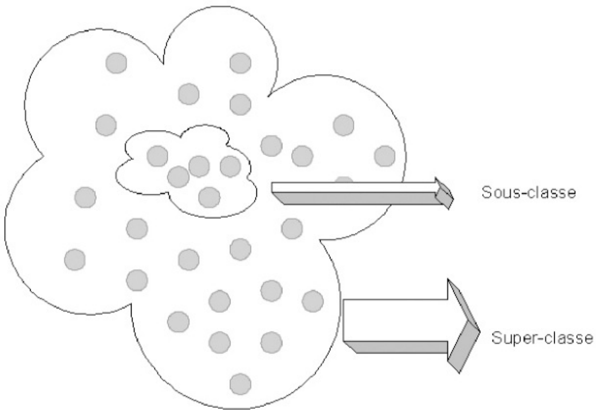
Figure 11-4 Interprétation ensembliste de l'héritage
