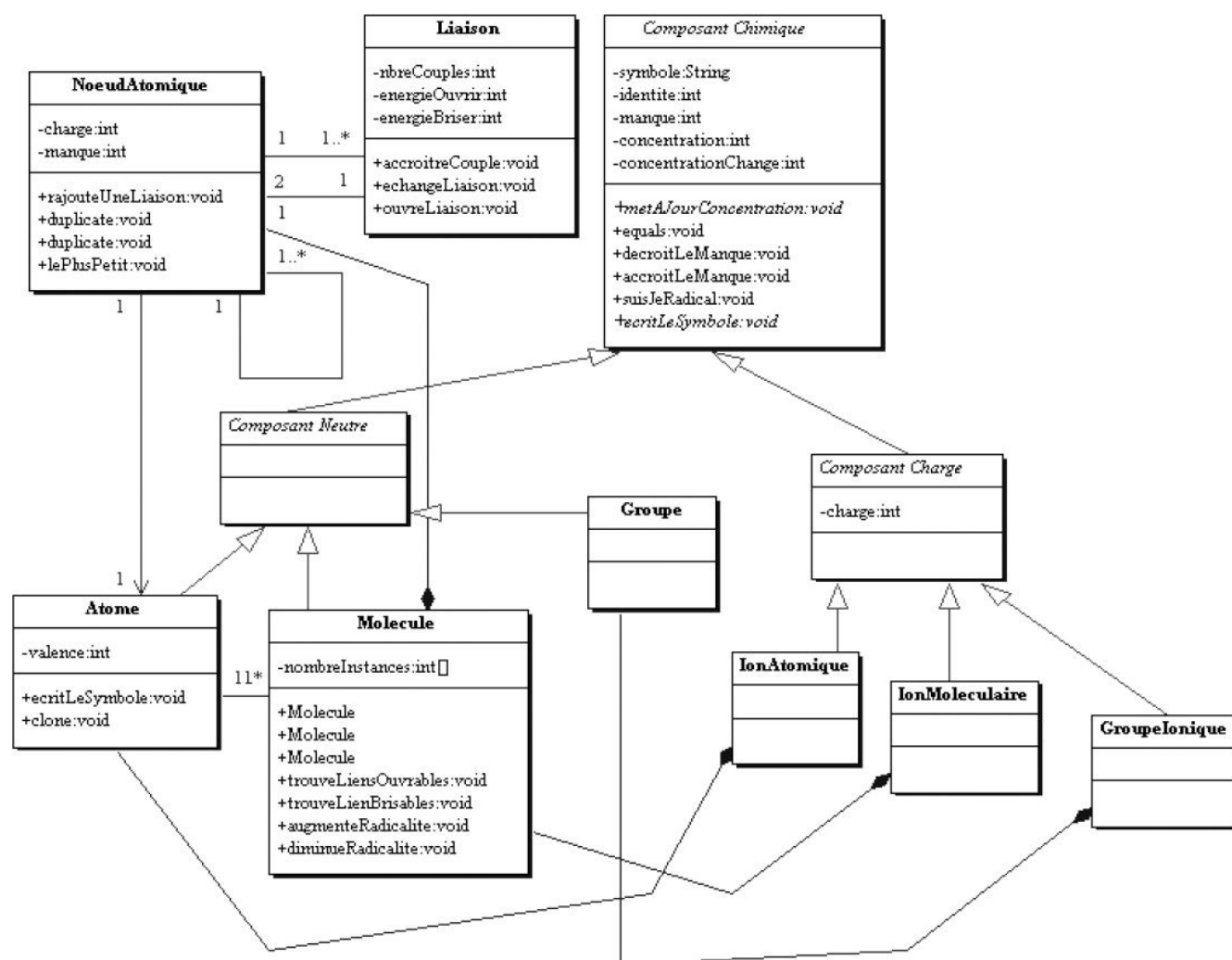
Figure 22–5 Version finale du diagramme de classes des éléments structuraux de notre réacteur chimique
