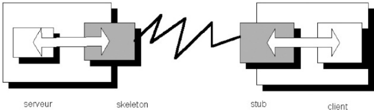
Figure 16–1 Les rôles joués par le stub et le skeleton
