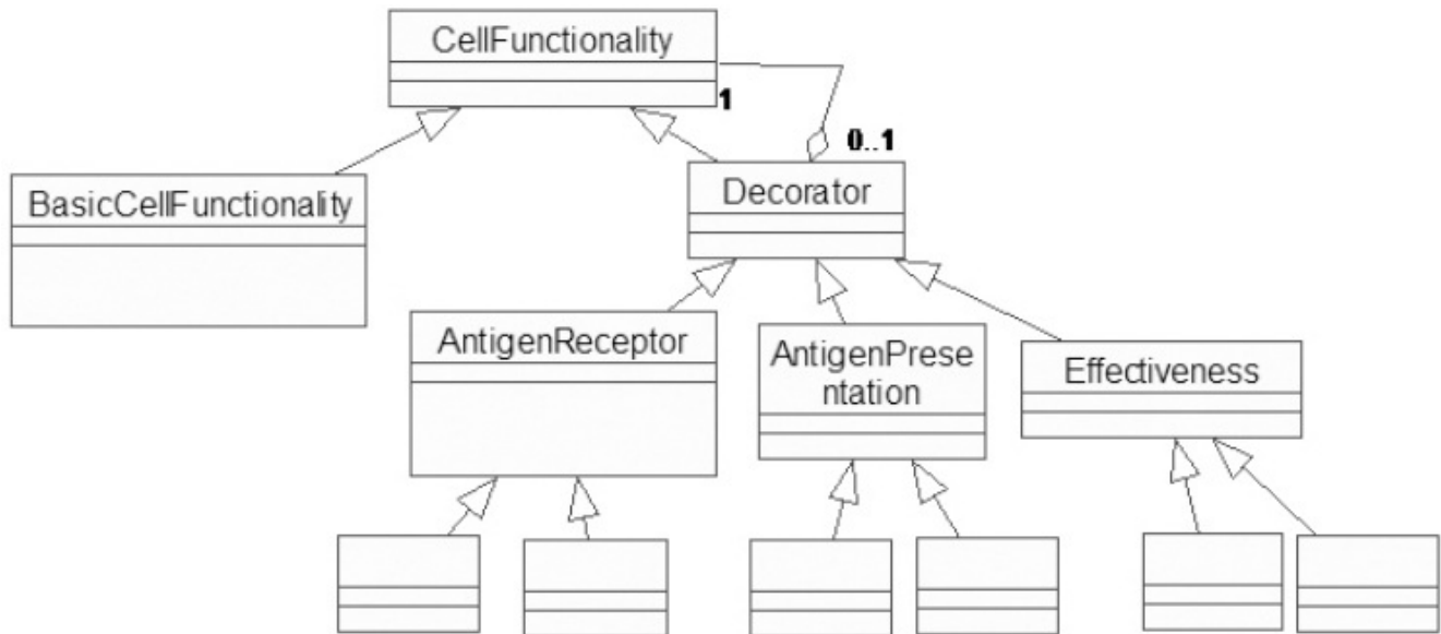
Figure 24-8 Le pattern Décorateur appliqué à l'immunologie
