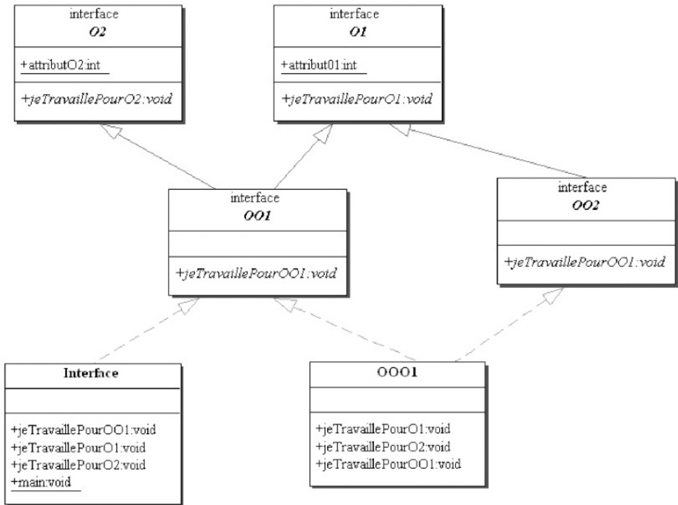
Figure 15–1 Structure d’héritage des interfaces. Dans ce diagramme de classes UML, figurent quatre interfaces (O2, O1, OO1 et OO2) et deux classes (OOO1 et Interface).
