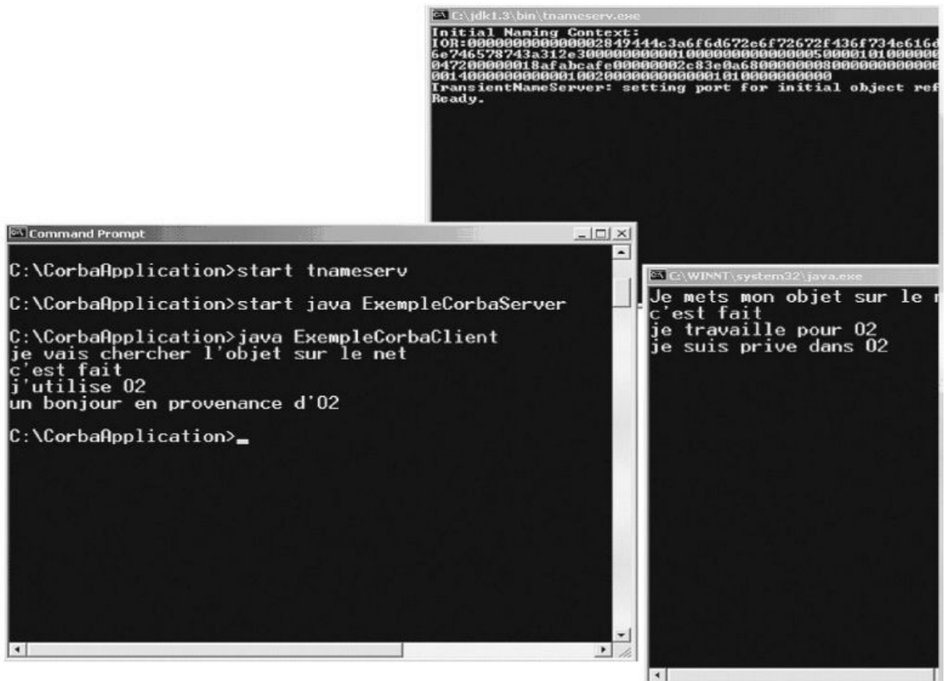
Figure 16–3 Déroulement de l'interaction Corb client-serveur en local et à partir d'une fenêtre d'invite de commande
