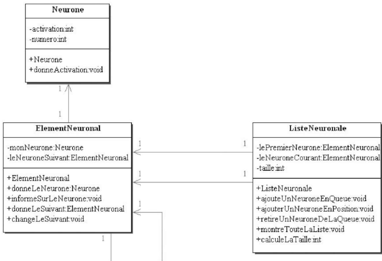
Figure 21-4 Diagramme de classes d'une liste liée
