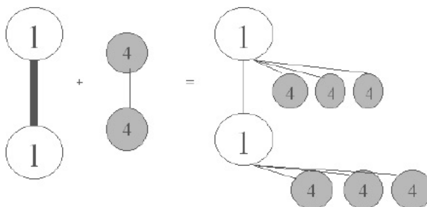
Figure 22–10 Illustration de la réaction d'ouverture de liaison : 1(1) + \{3 \times\} 4(4) \leftrightarrow 1(1(444)444)
