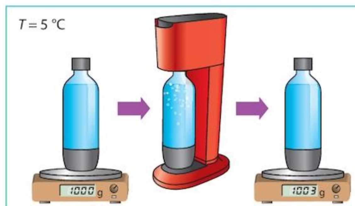
FIG. 2b Masse maximale de 1 L d'eau gazéifiée obtenue avec de l'eau fraîche
