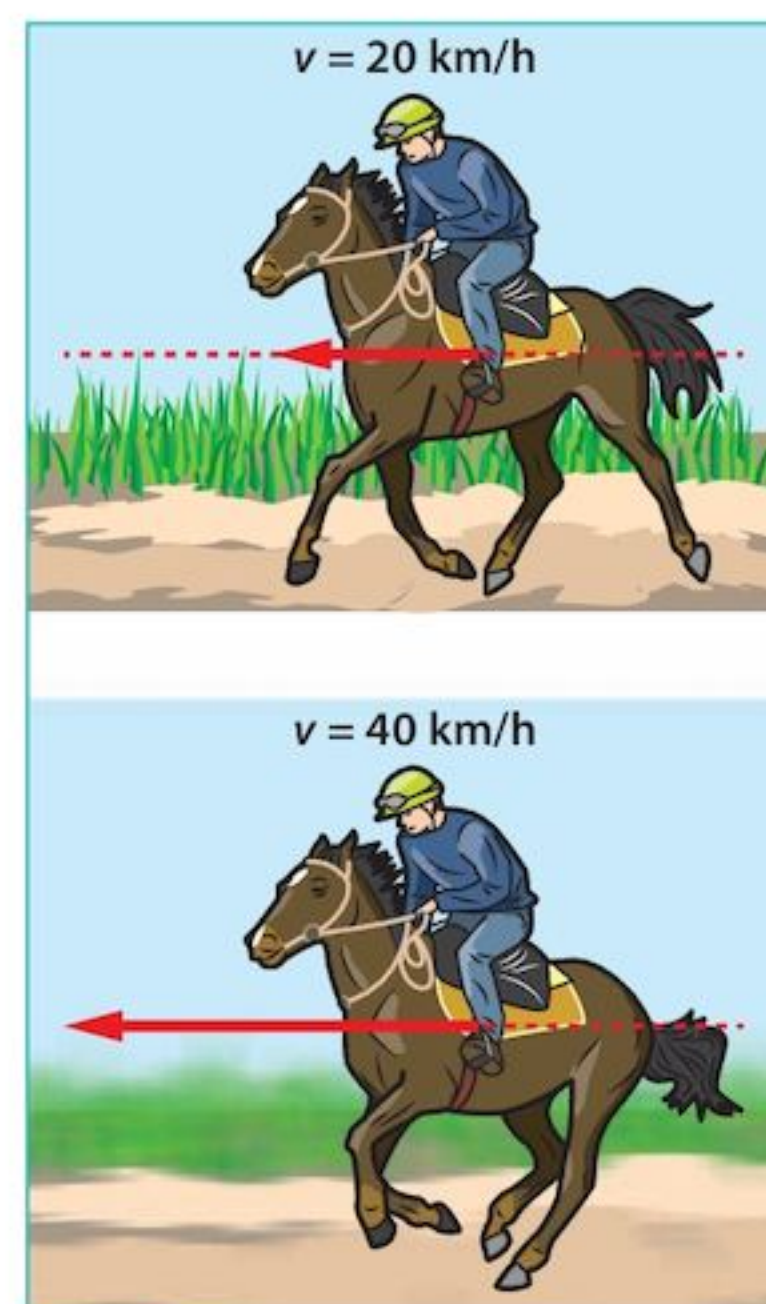
FIG. 2 Représentation de la vitesse d'un cheval
