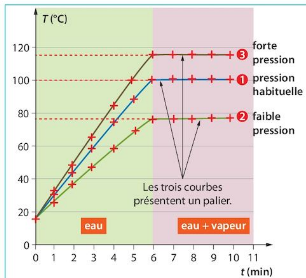
FIG. 2 Courbes d'ébullition de l'eau pure
