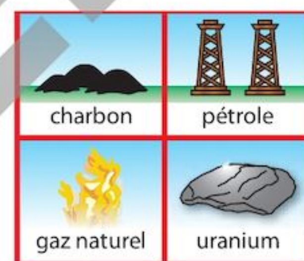
FIG. 1b Sources d'énergie non renouvelables
