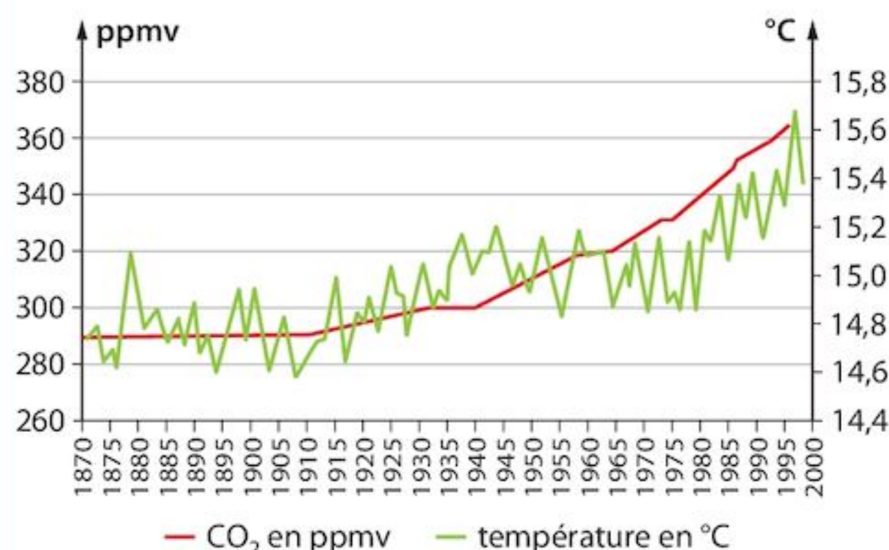
Évolution comparée de la teneur en CO 2 et de la température moyenne de l'atmosphère
