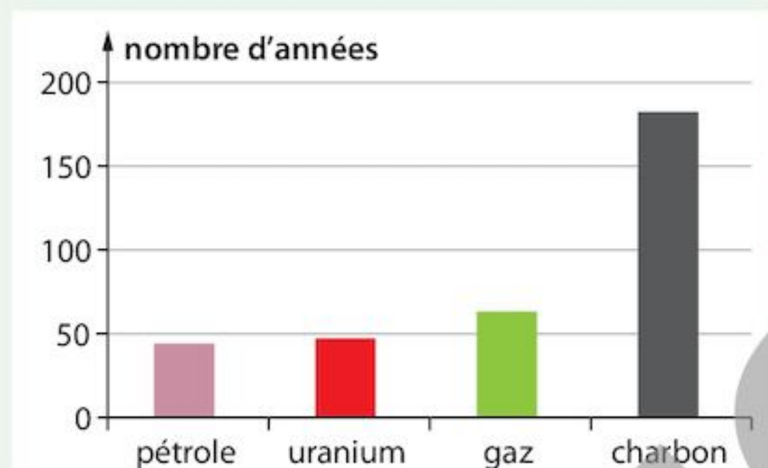
FIG. 1 Estimation des réserves mondiales d'énergie (d'après BP Statistical Review of World Energy, 2009)
