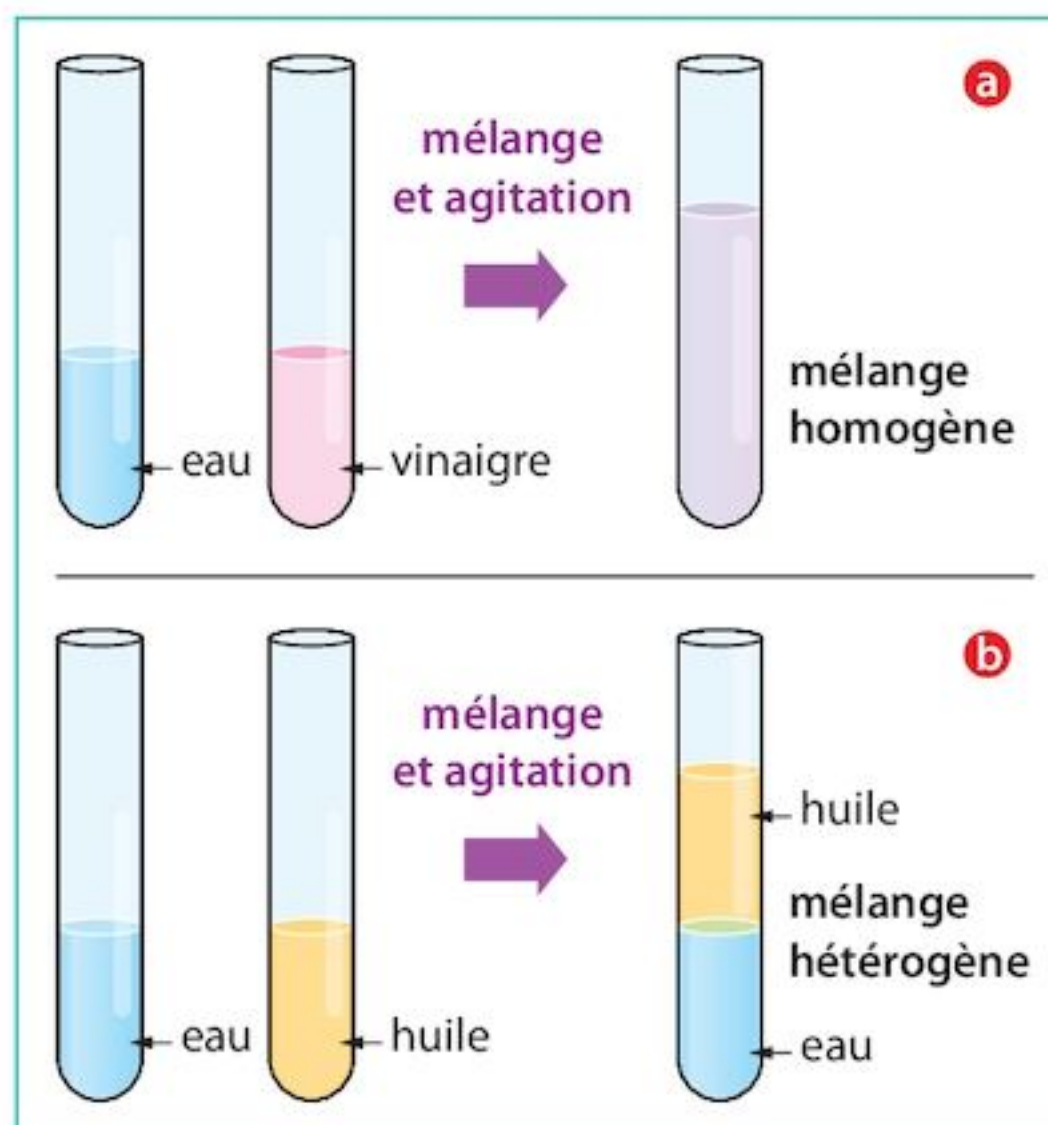
FIG. 2 Miscibilité des liquides avec l'eau
