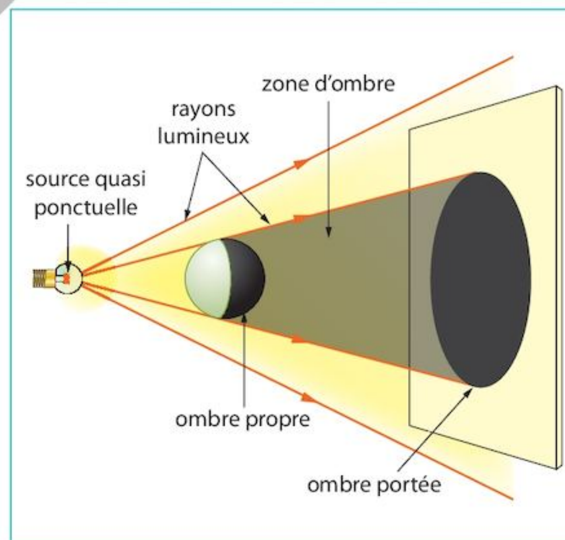
FIG. 2 Ombres formées par un faisceau lumineux
