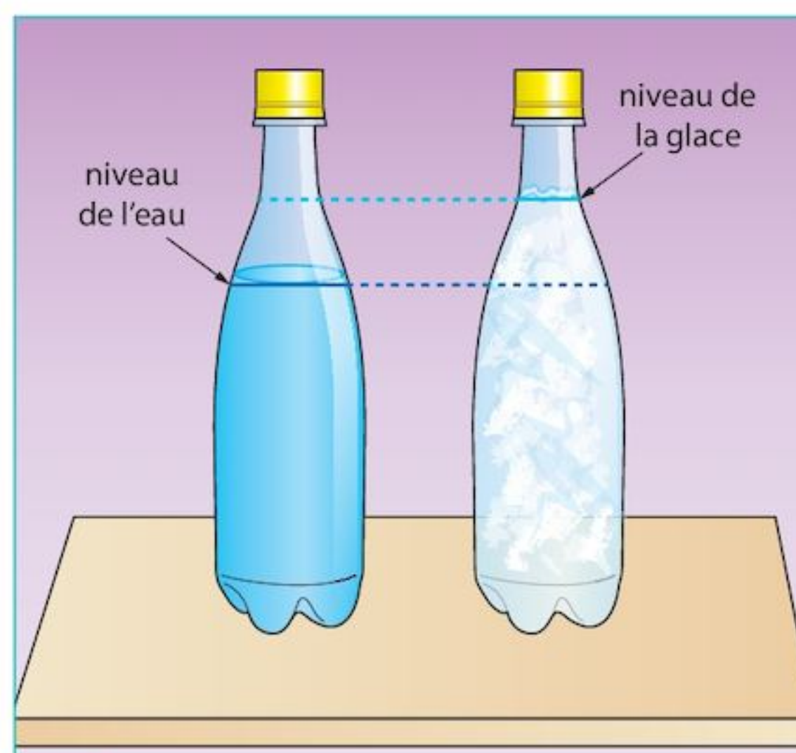
FIG. 2 Solidification de l'eau
