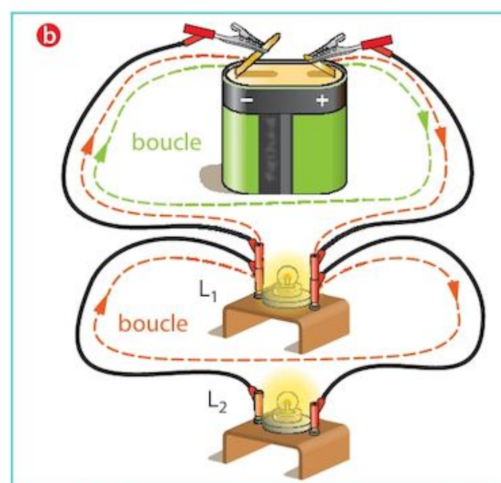
FIG. 2 Dipôles en série a et en dérivation b
