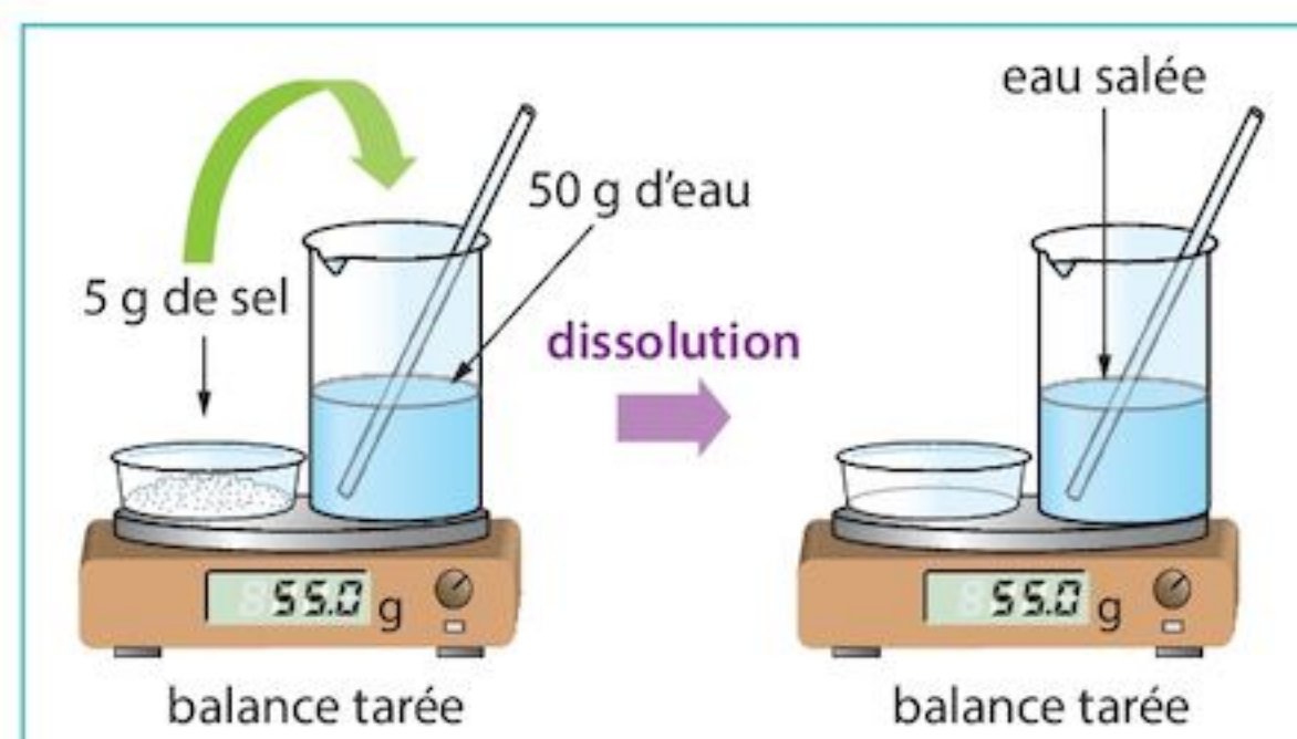
FIG. 3 Dissolution du sel dans l'eau
