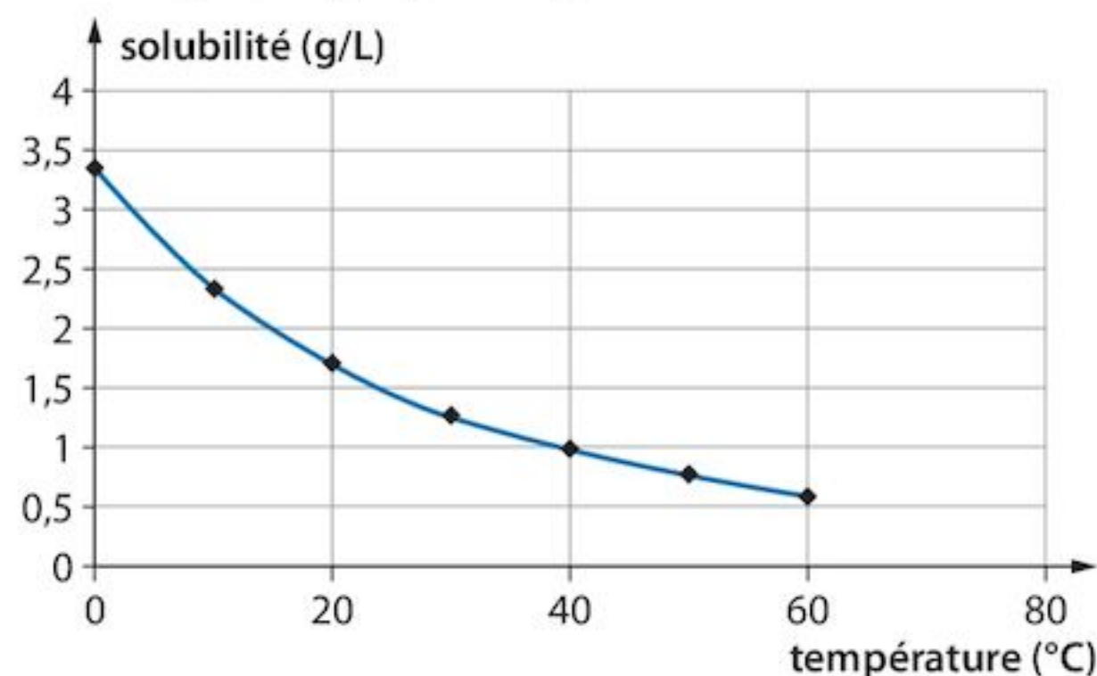
Solubilité du dioxyde de carbone dans l'eau
