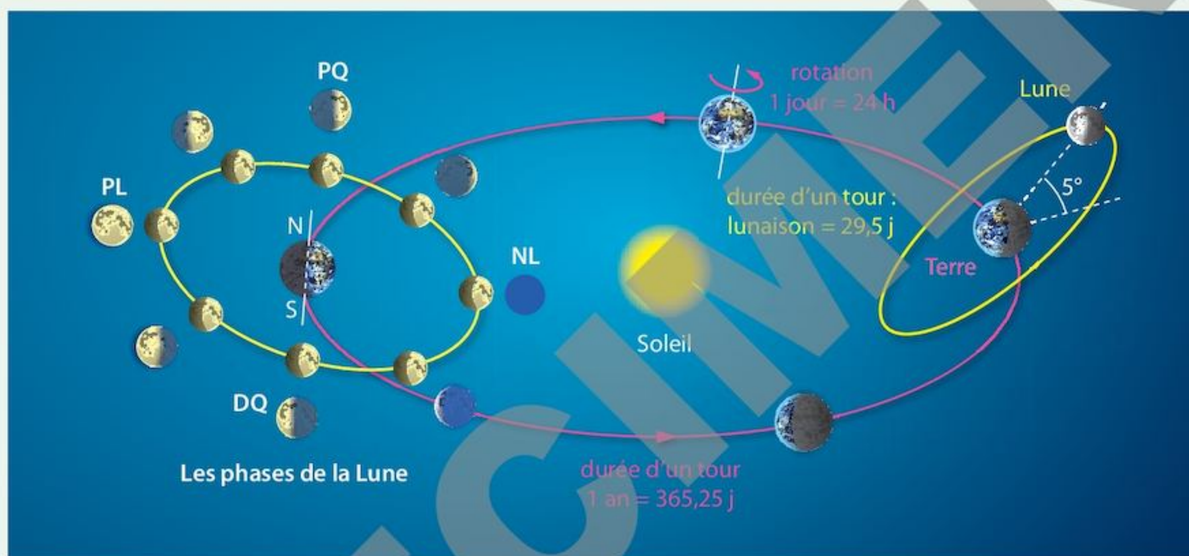
FIG. Mouvements de la Terre et de la Lune
