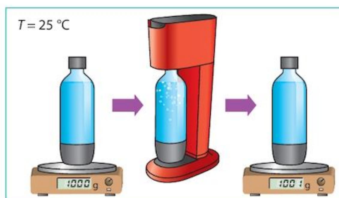
FIG. 2a Masse maximale de 1 L d'eau gazéifiée obtenue avec de l'eau tiède
