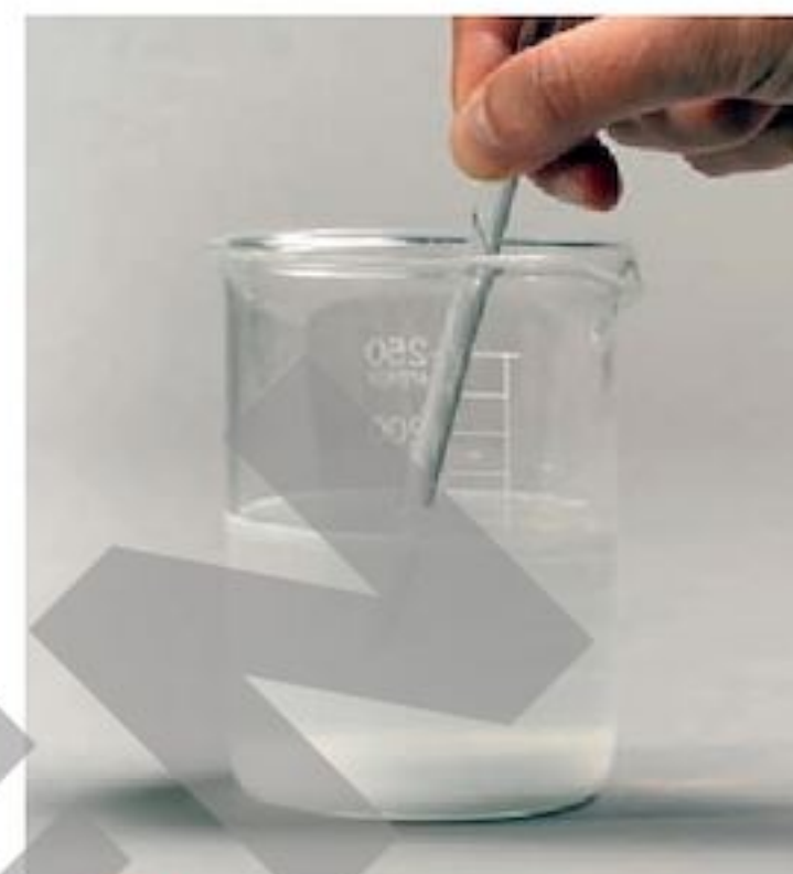
FIG. 3 Après ajout de suffisamment de sel
