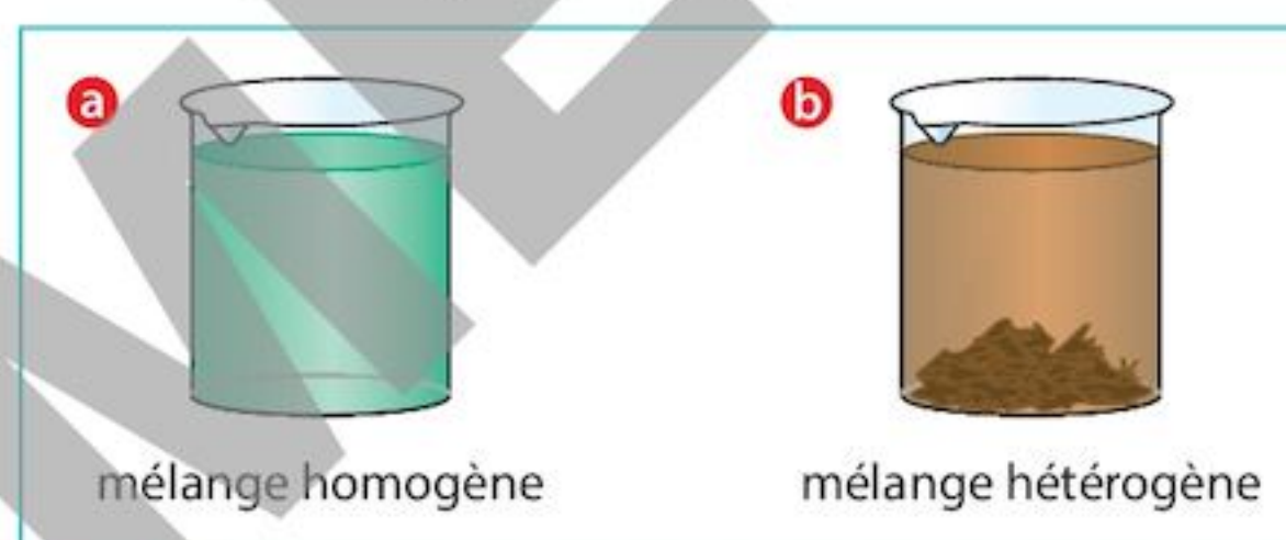
FIG. 2 Exemples de mélanges homogène et hétérogène
