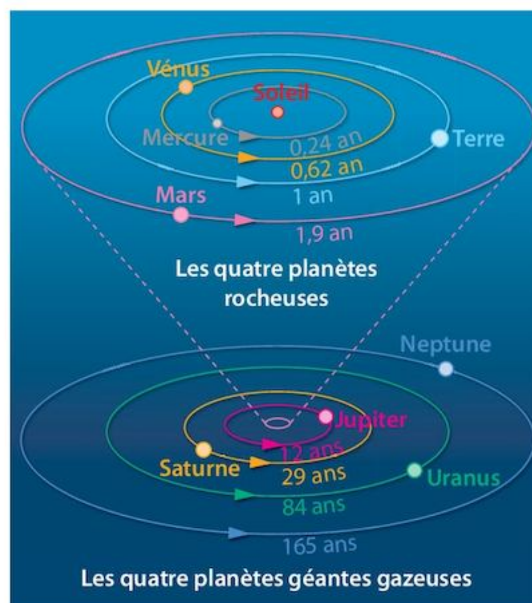
FIG. 2 Les planètes du système solaire
