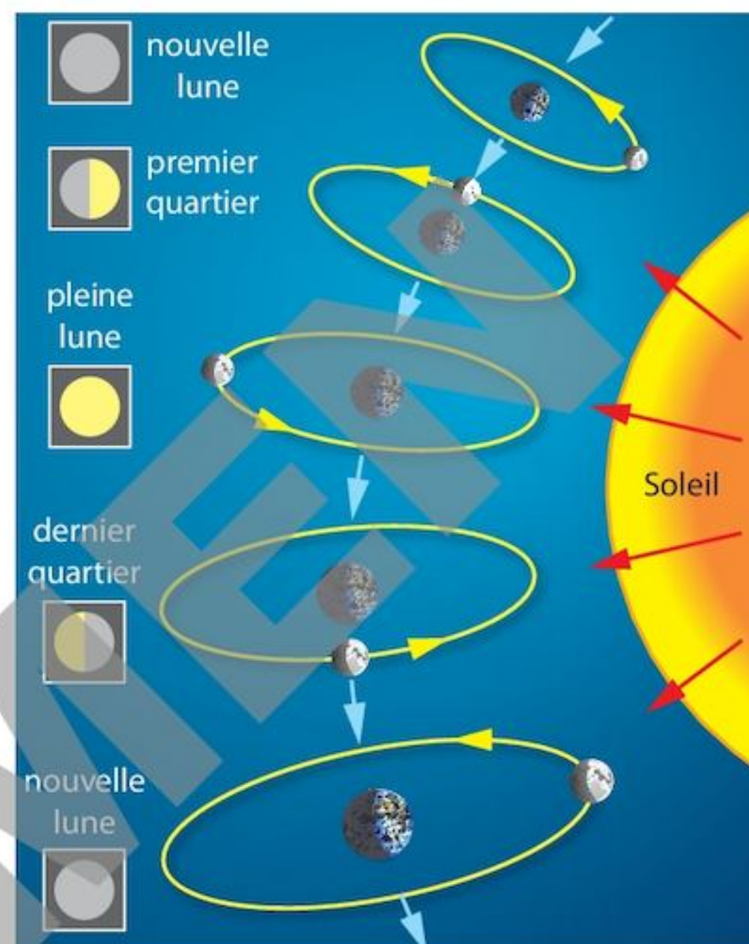
FIG. 1 Mouvements de la Terre et de la Lune
