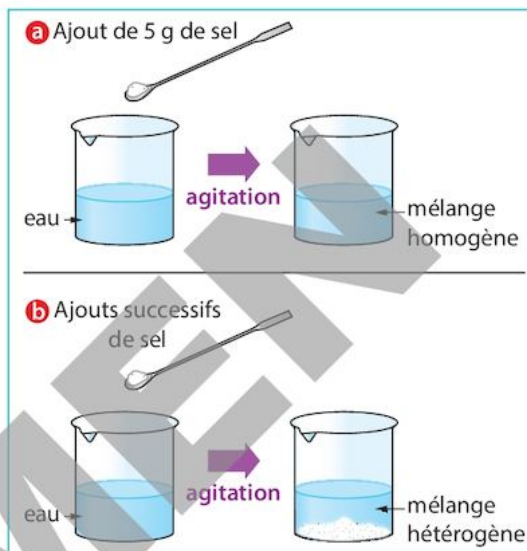
FIG. 1 Dissolution du sel dans l'eau
