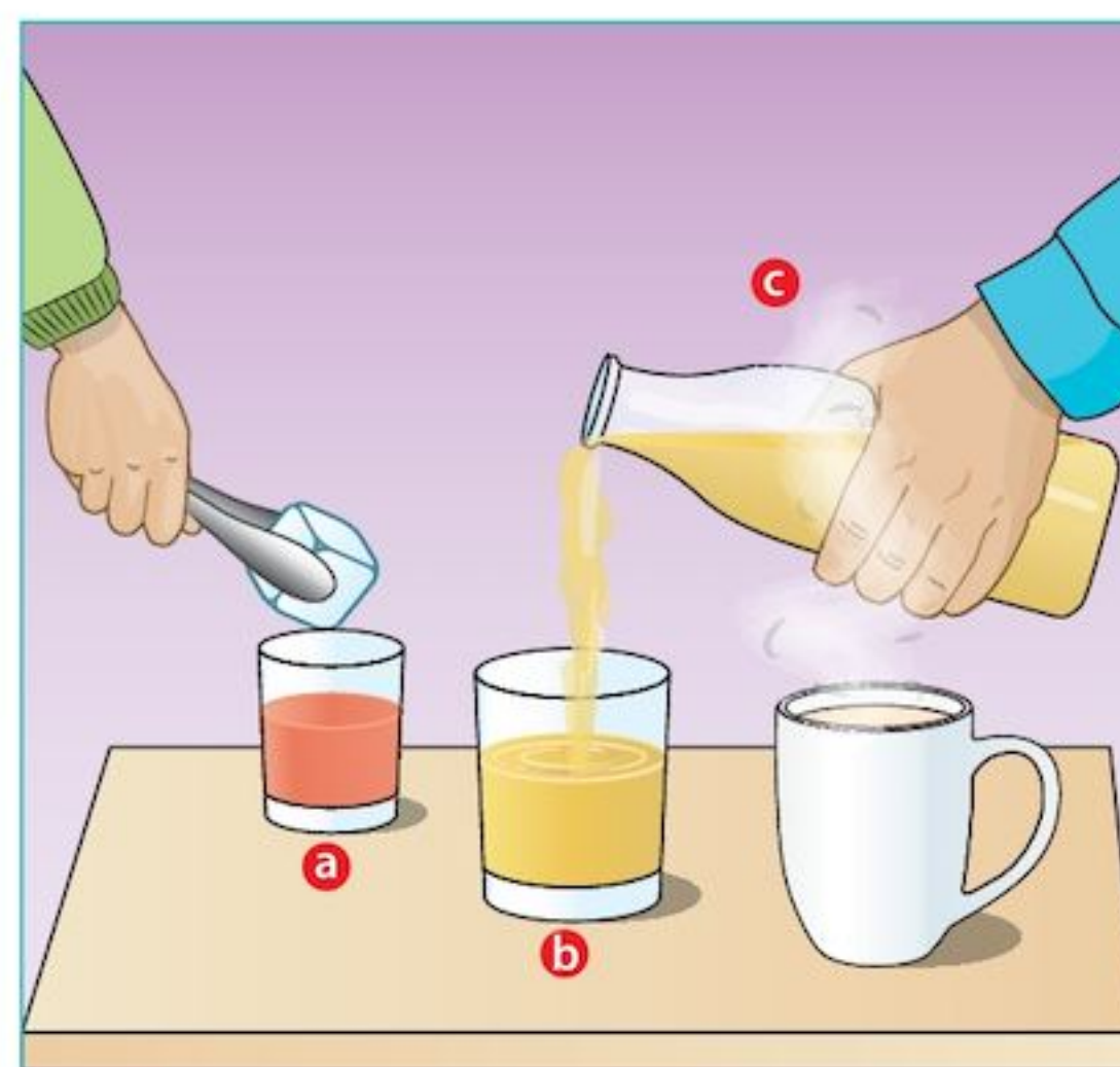
FIG. 2 Les propriétés des états de l'eau
