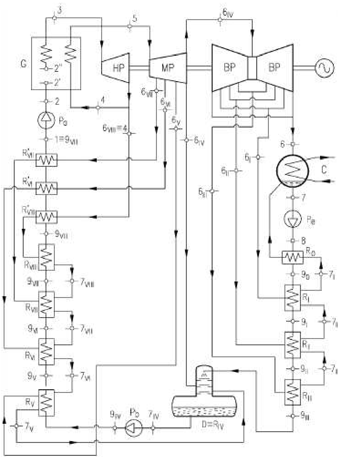
FIG. VI.6 – Cycle complexe d'une turbine à vapeur
