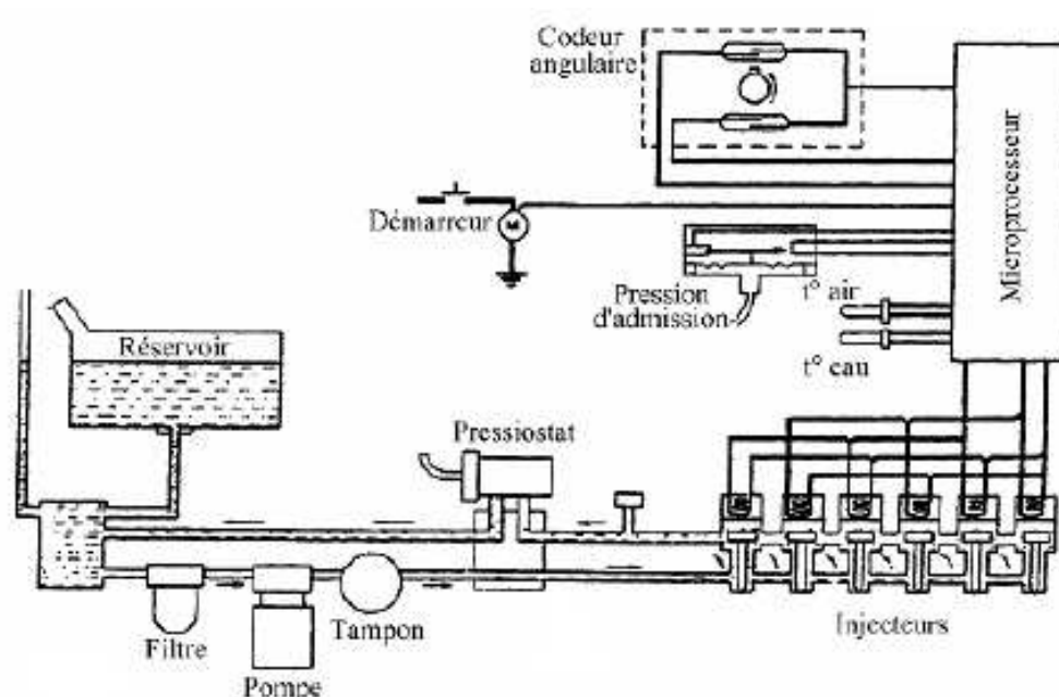
FIG. V.3 – Schéma système d'injection moteur essence
