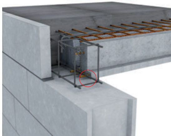
Pour les poutrelles : l'appui minimal sur mur en maçonnerie est de 5 cm
