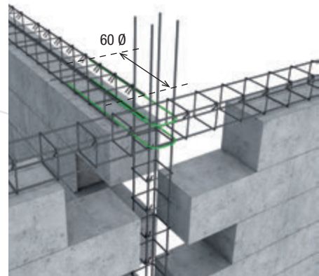
Liaison en partie courante avec boucles
