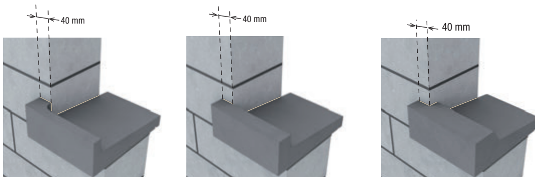
Rejingot sans feuillure
