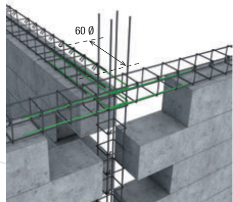
Liaison en partie courante avec équerres
