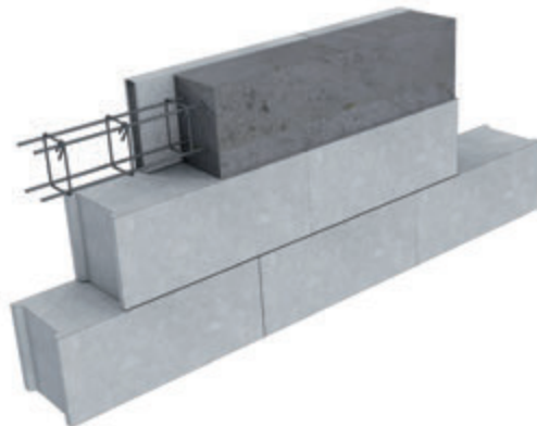
Détail des chaînages en situation sismique. Ouverture de 15 cm
