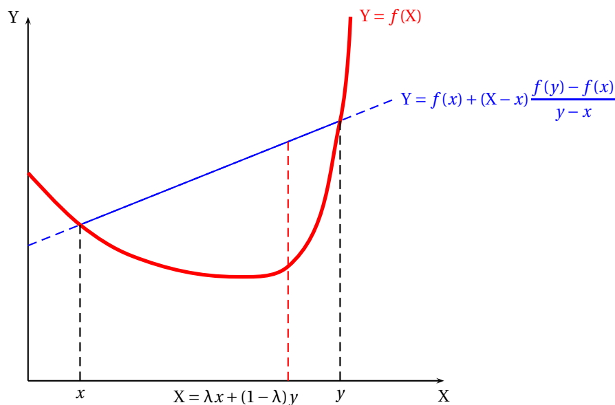
FIGURE 12.6 – Fonctions convexes
