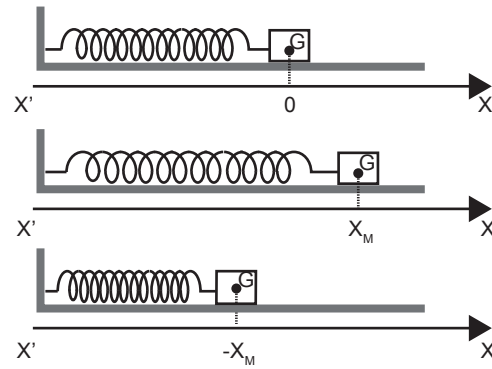
Pendule élastique horizontal
