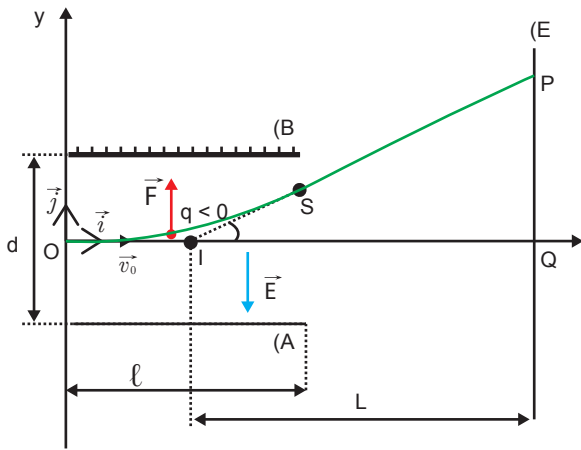
Mouvement d'une particule chargée dans un champ électrostatique
