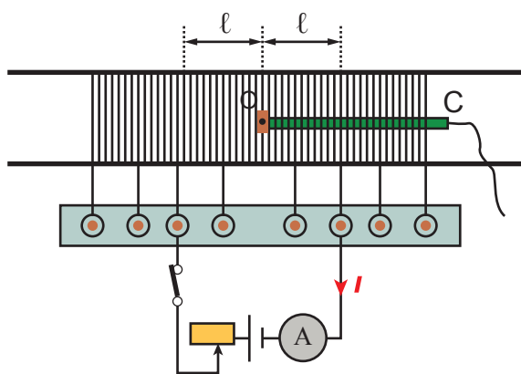
Mesure de la valeur du champ magnétique à l'intérieur d'un solénoïde
