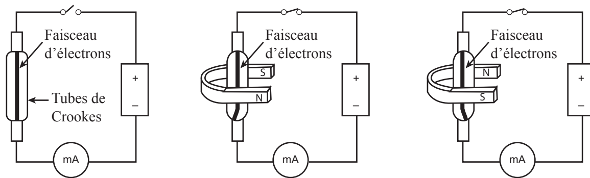
Action d'un aimant en U sur un faisceau d'électrons en mouvement
