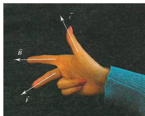
Utilisation de la règle des trois doigts la main droite
