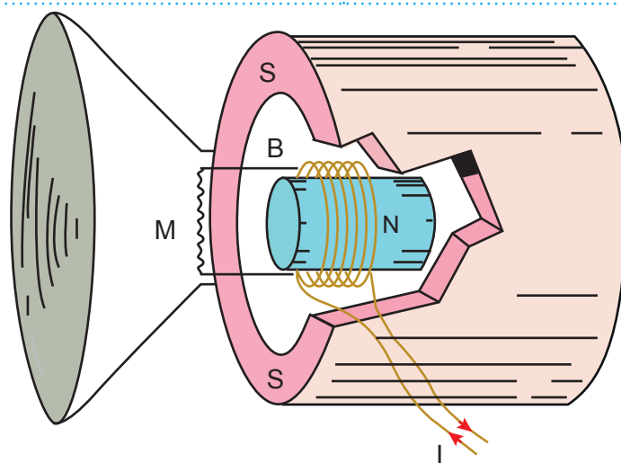
Coupe d'un haut-parleur
