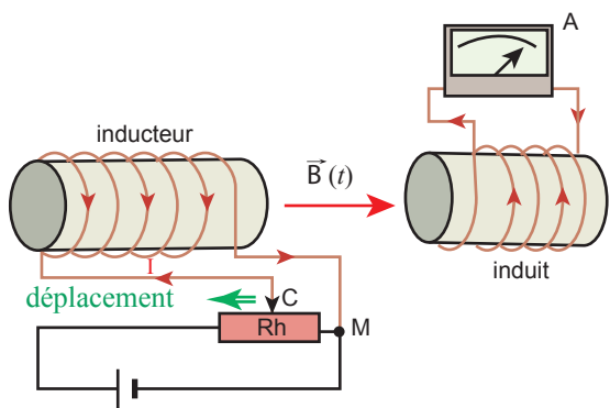
Déplacement d'une bobine parcourue par un courant par rapport à une autre bobine
