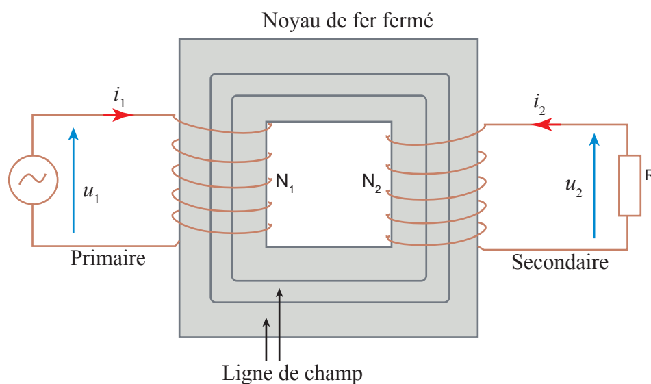
Schéma d'un transformateur
