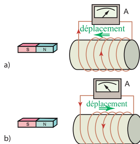
Déplacement d'une bobine par rapport à un aimant
