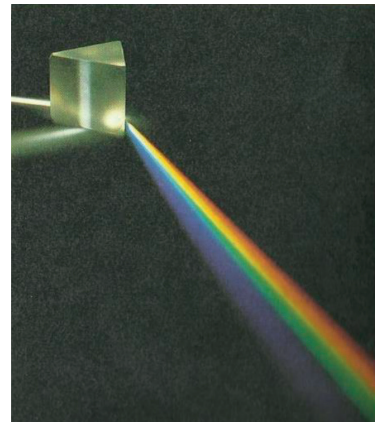
Décomposition de la lumière blanche par un prisme
