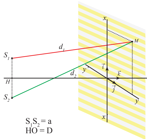
Schéma de l'expérience des trous d'YOUNG
