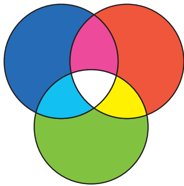
Synthèse de la lumière blanche
