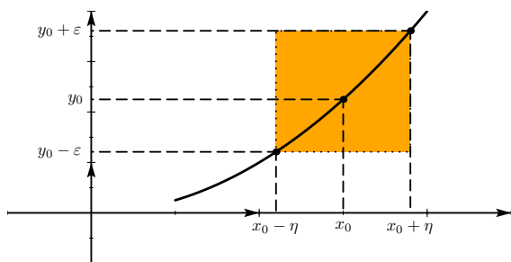
FIGURE 11.1 – Avec \varepsilon = 0.4
