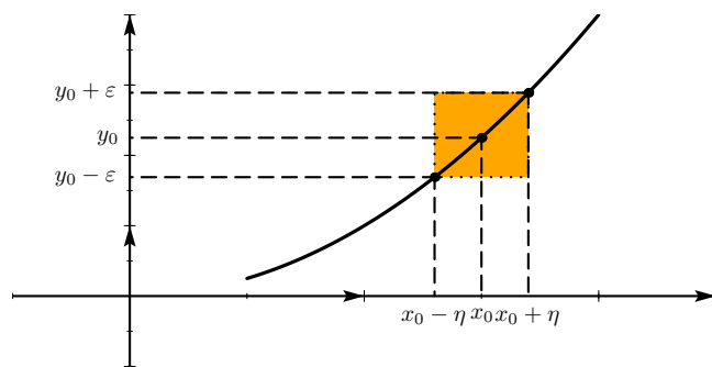
FIGURE 11.2 – Avec \varepsilon = 0.2
