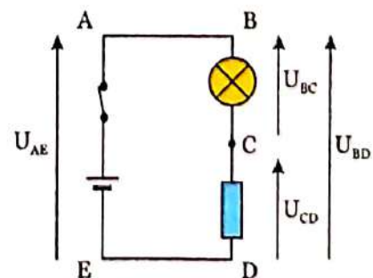
Doc. 5 Additivité des tensions.
