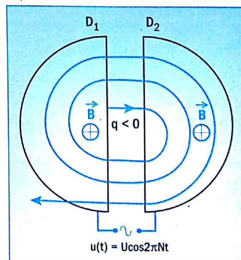
Fig. 11. Le cyclotron
