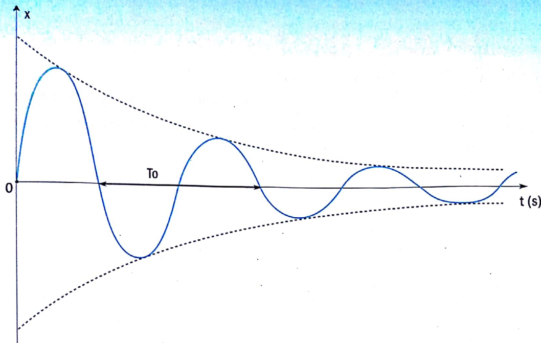
Fig. 5. Oscillations amorties. Le mouvement est pseudo-périodique.
