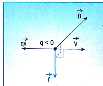
Fig. 6. Force de Lorentz s'exerçant sur un électron
