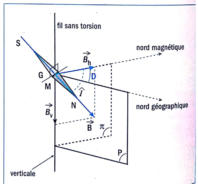
2. En France, le champ magnétique terrestre \vec{B} plonge vers le sol. - D : angle de déclinaison ; à Paris : D = 5,5^\circ - I : angle d'inclinaison ; à Paris : I = 64,5^\circ - B_h composante horizontale du champ magnétique terrestre ; actuellement B_h = 2,10^{-5}\text{ T} ; B_h est dirigé vers l'ouest.
