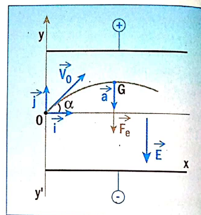
Fig. 11. Z = 0 , le mouvement se fait dans le plan (xOy)
