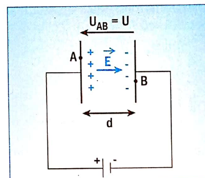
Fig. 9. Champ électrostatique uniforme
