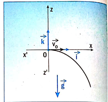
Fig. 5. Arc de parabole
