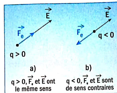
Fig. 8. Force électrique
