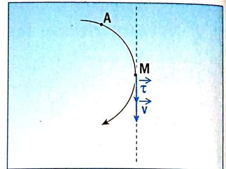
Fig. 7. Vecteur vitesse \vec{v} dans le repère (M, \vec{\tau}) , \vec{v} = v\vec{\tau} .
