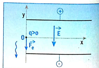
Fig. 12. Mouvement rectiligne uniformément accéléré
