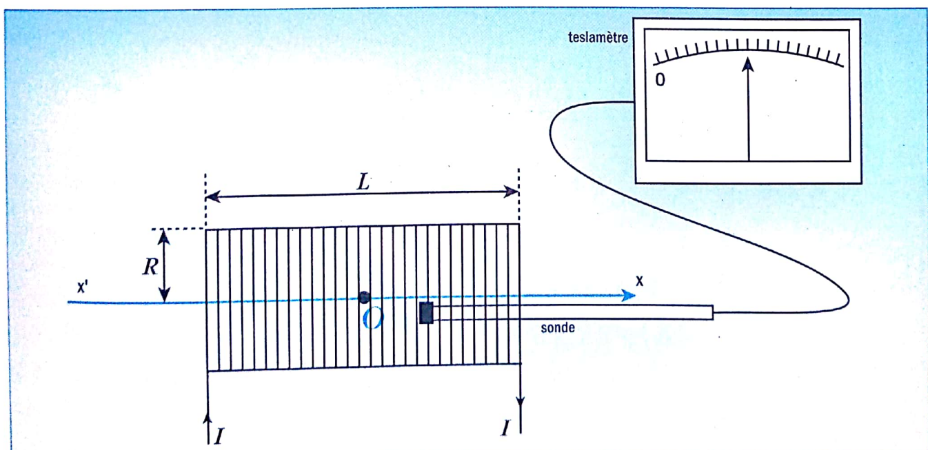
Fig. 18. Mesure de la valeur du champ magnétique à l'intérieur d'un solénoïde
