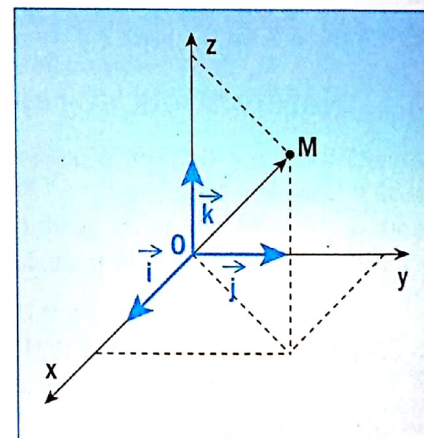
Fig. 3. Vecteur position \vec{OM} = x\vec{i} + y\vec{j} + z\vec{k}
