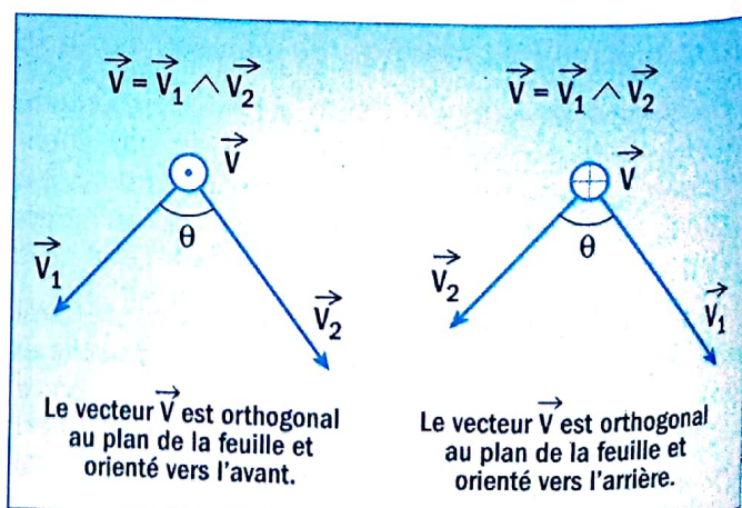
Fig. 2. Convention de représentation des vecteurs
