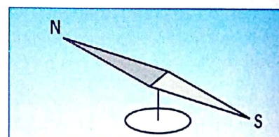
Fig. 1. Une aiguille aimantée
