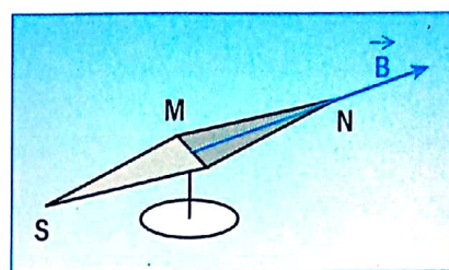
Fig. 4. Vecteur champ magnétique au point M, analysé à l'aiguille aimantée
