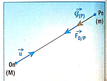
Fig. 2. Vecteur champ de gravitation
