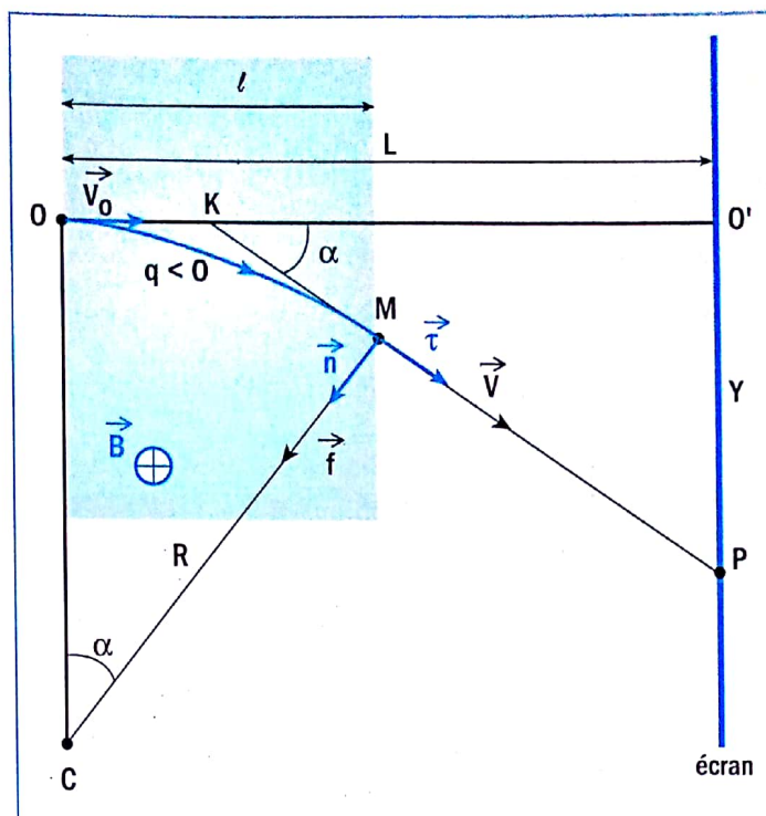
Fig. 10. La déflexion magnétique
