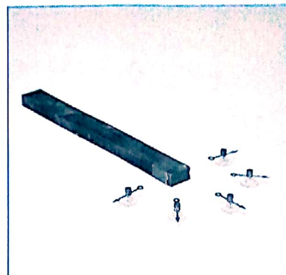
Fig. 3. Champ magnétique d'un aimant droit *
