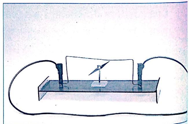
Fig. 9. L'expérience d'Ørsted *
