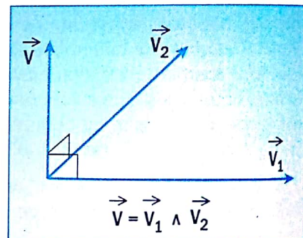
Fig. 1. Le produit vectoriel de deux vecteurs
