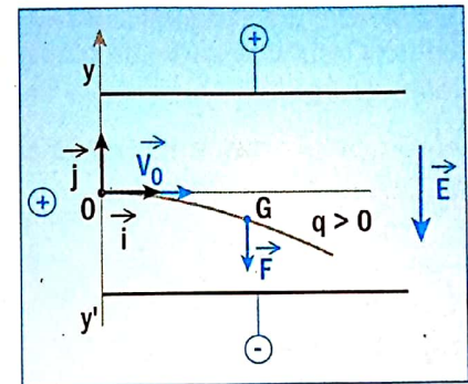
Fig. 14. ( \vec{V}_0 \perp \vec{E} ), la trajectoire est parabolique
