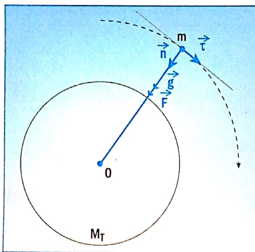
Fig. 6. Mouvement circulaire d'un satellite
