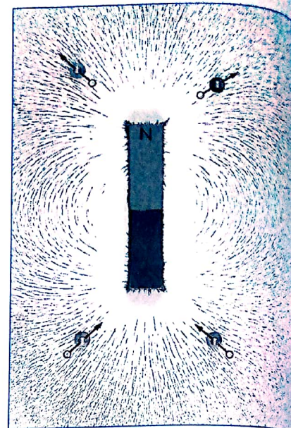
Fig. 14. Spectre magnétique d'un aimant droit *
