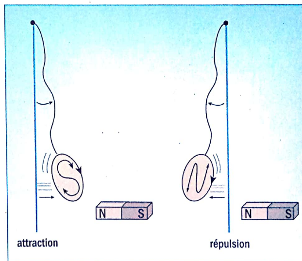
Fig. 12. Interaction aimant-courant
