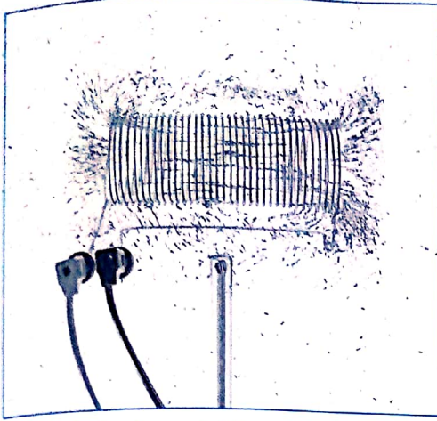
Fig. 17-1. Spectre magnétique d'un solénoïde *
