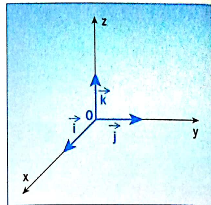
Fig. 2. Exemple de repère d'espace
