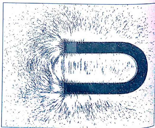
Fig. 16. Lignes de champ d'un aimant en U *
