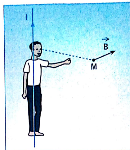
Fig. 10. Règle de l'observateur ou bon-homme d'Ampère
