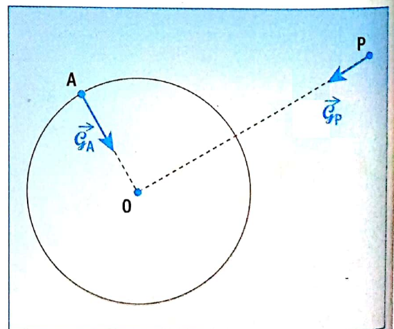
Fig. 3. Champ de gravitation créé par un solide à répartition sphérique de masse
