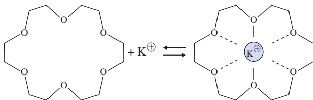
éther - 18 couronne - 6
