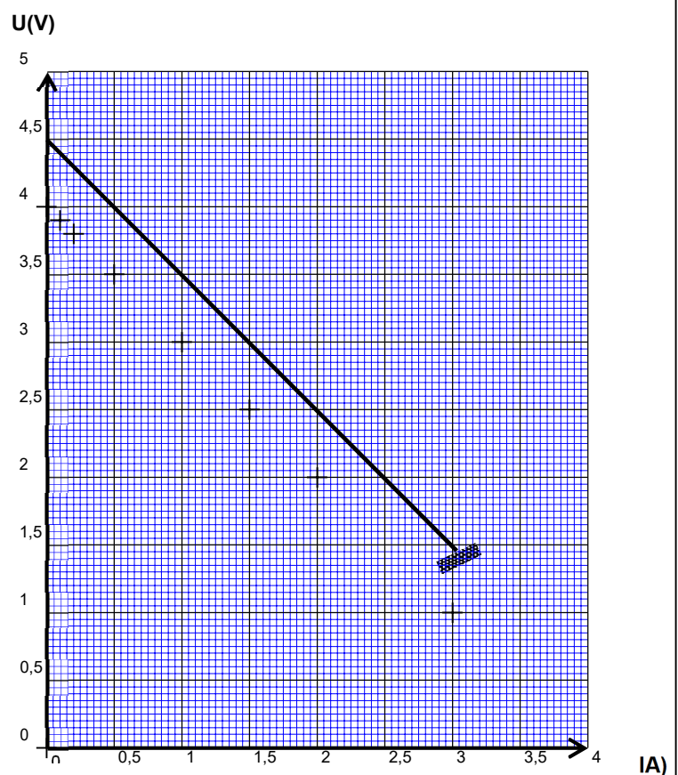
Figure 2 : Caractéristique U = f(I)
