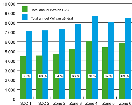
Figure 23 Pourcentage de la consommation énergétique des CVC par rapport à la consommation énergétique totale suivant les zones climatiques du Maroc
