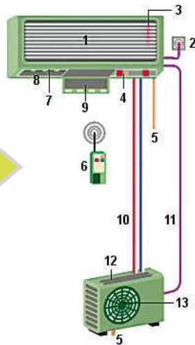
Figure 6 Unité extérieure et intérieure d'un climatiseur individuel de type split système
