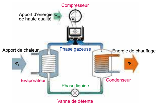
Figure 3 Schéma de principe d'une pompe à chaleur en mode chauffage
