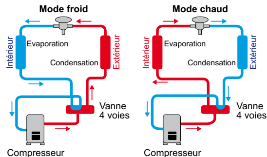
Figure 5 Pompe à chaleur réversible
