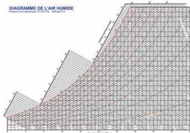
Figure 27 Diagramme psychrométrique pour l'air humide
