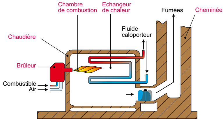
Figure 2 Coupe schématique d'une chaudière (source : énergétique du bâtiment, Claude-Alain Roulet)
