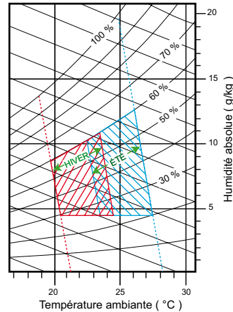
Figure 25 Plages de confort hygrothermiques pour des activités de bureau
