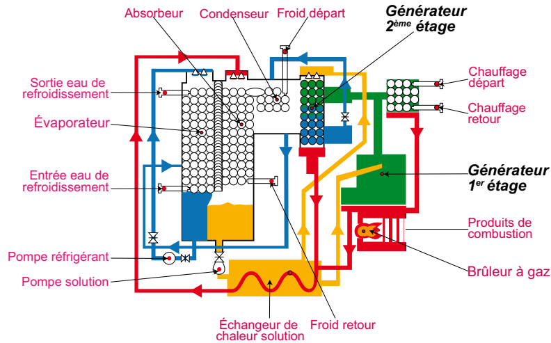
Figure 10 Cycle typique d'un refroidisseur à absorption à combustion directe
