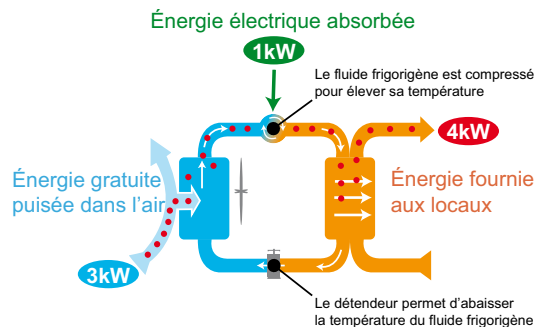
Figure 4 Transfert d'énergie d'une PAC en mode chauffage
