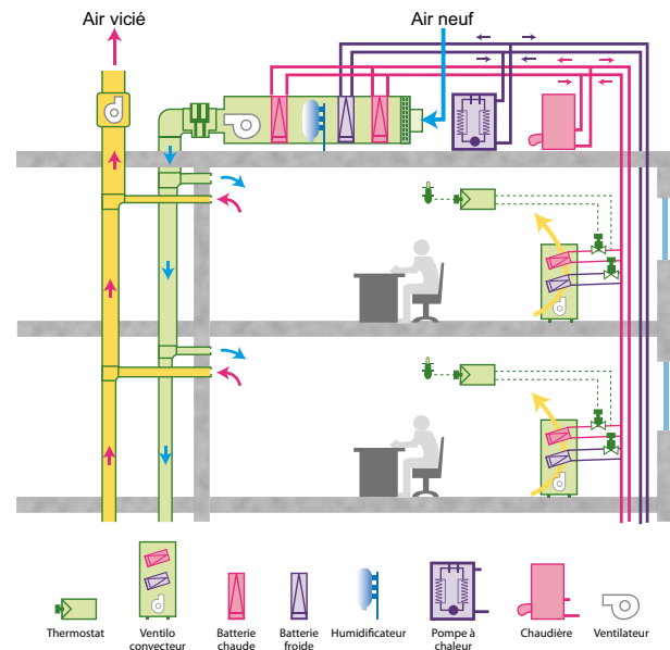
Figure 17 Schéma général d'un système CVC centralisé
