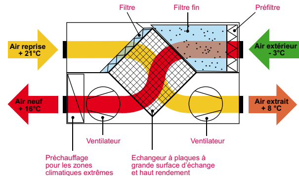
Figure 11 Schéma de fonctionnement d'une ventilation double flux à échangeur thermique
