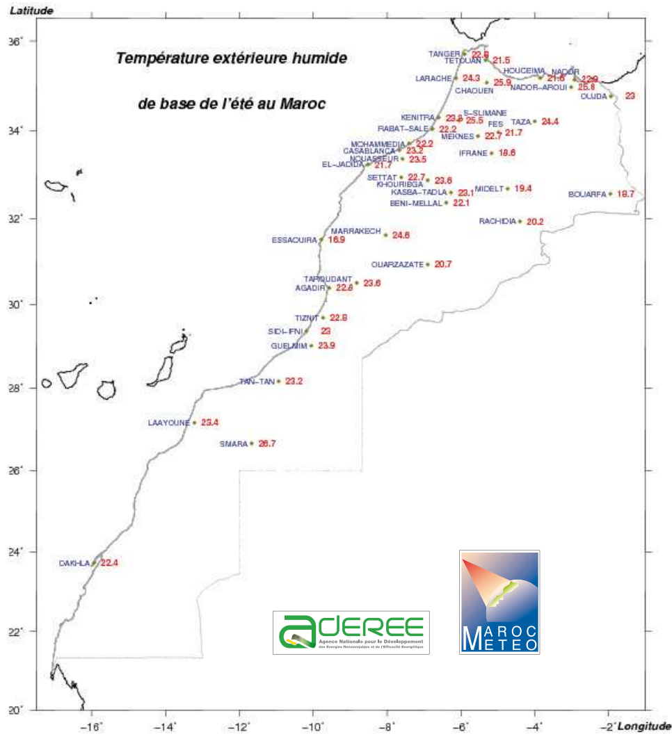
Figure 30 Carte des 38 stations météorologiques et leurs températures humides de base de l'été
