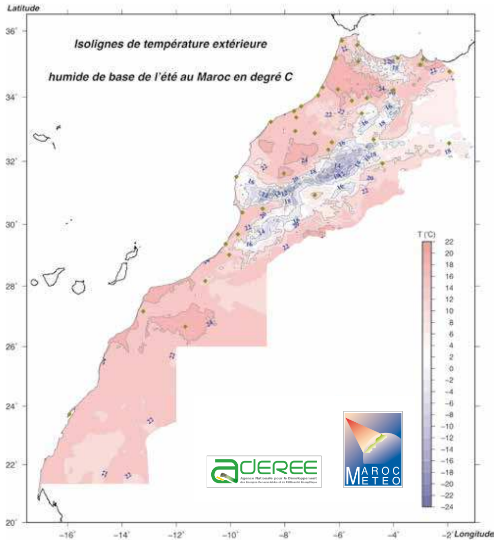
Figure 34 Carte des iso-températures extérieures humides de base de l'été calculées en se basant sur la correction par rapport à l'altitude.
