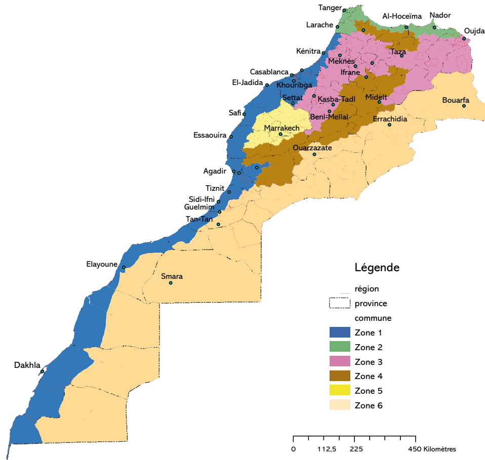
Figure 28 Carte du zonage climatique au Maroc adapté aux besoins du RTCM
