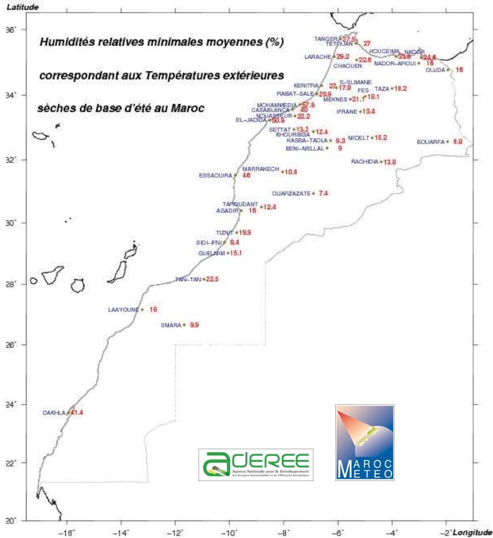
Figure 32 Carte des humidités relatives minimales moyennes correspondant aux températures extérieures sèches de base de l'été.
