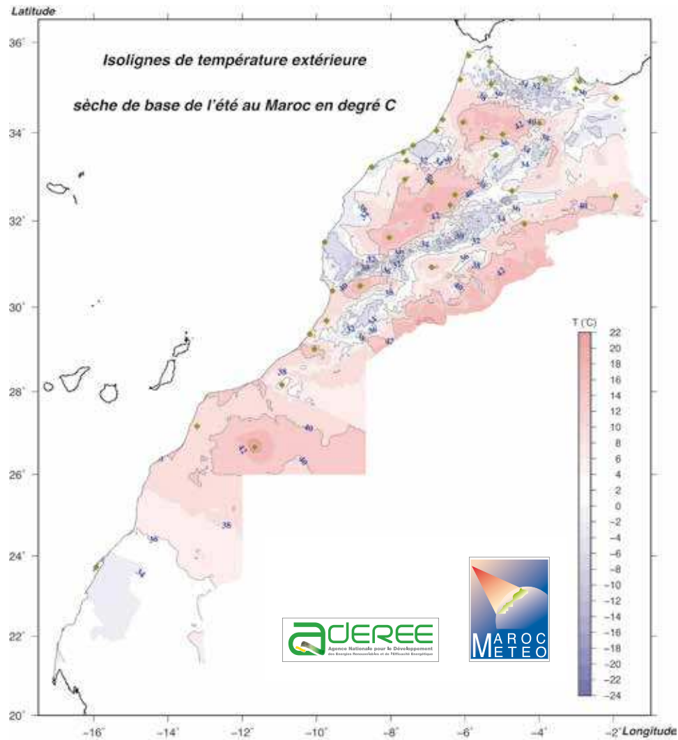
Figure 33 Carte des iso-températures extérieures sèches de base de l'été calculées en se basant sur la correction par rapport à l'altitude.
