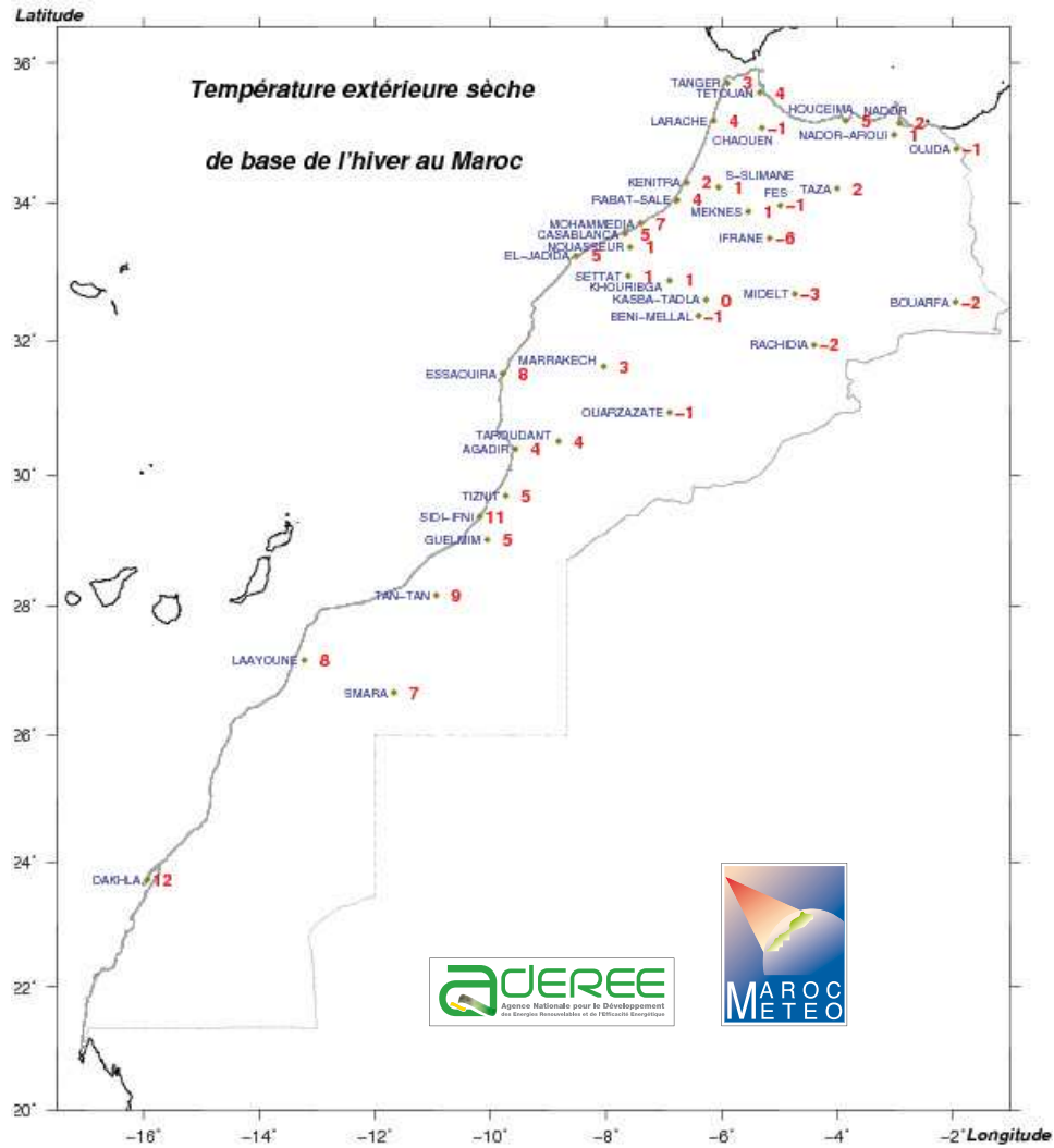
Figure 31 Carte des 38 stations météorologiques et leurs températures sèches de base de l'hiver
