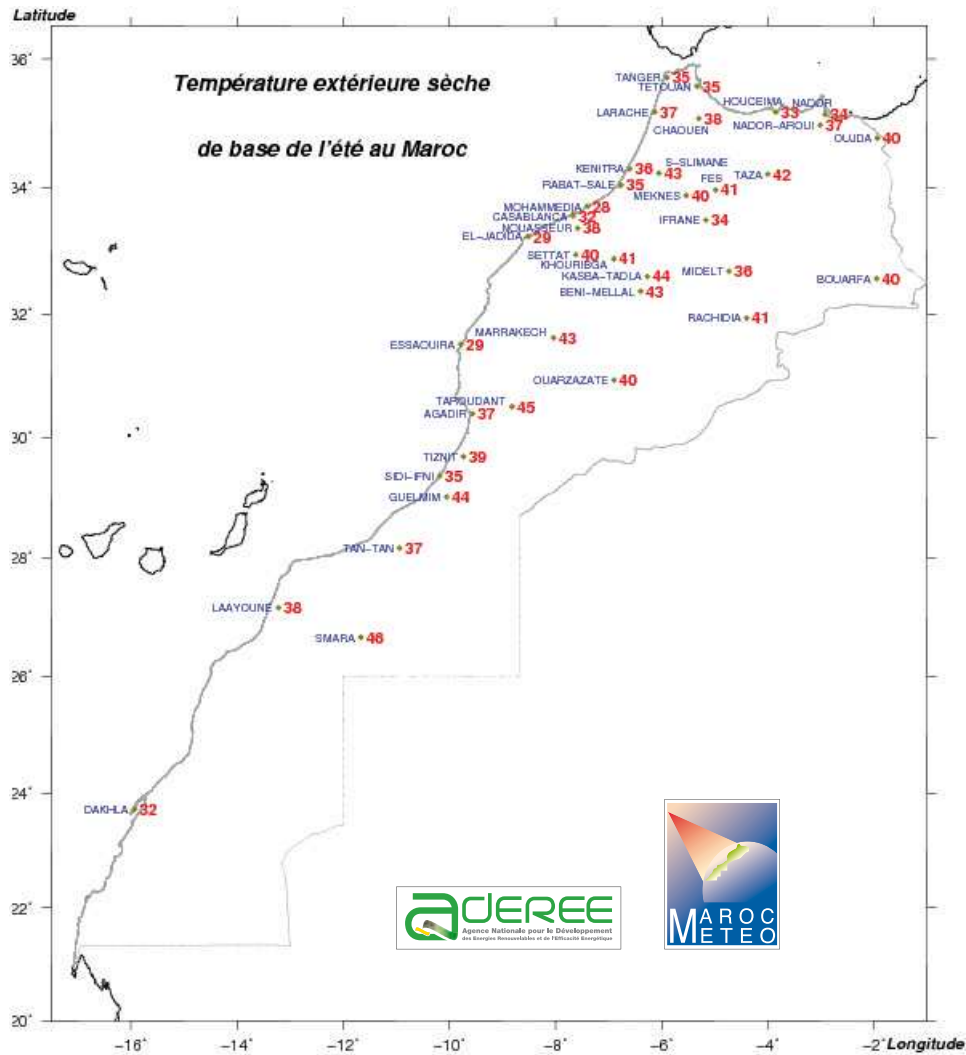
Figure 29 Carte des 38 stations météorologiques et leurs températures sèches de base de l'été
