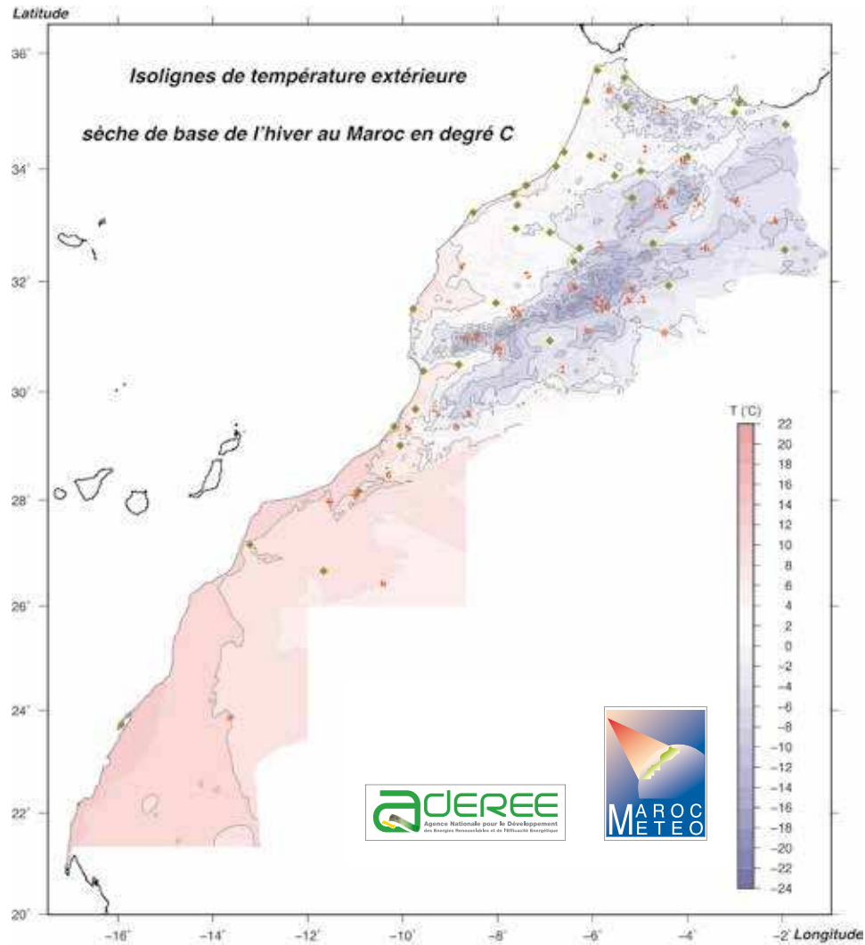
Figure 35 Carte des iso-températures extérieures sèches de base de l'hiver calculées en se basant sur la correction par rapport à l'altitude.
