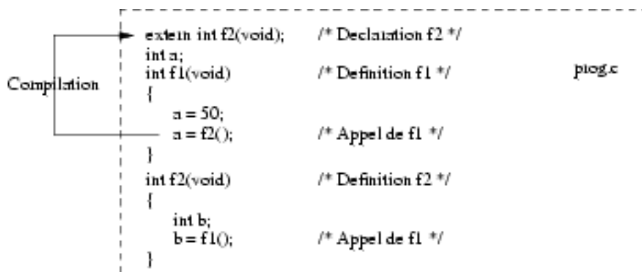
FIG. 9.6 – Visibilité des fonctions dans un module
