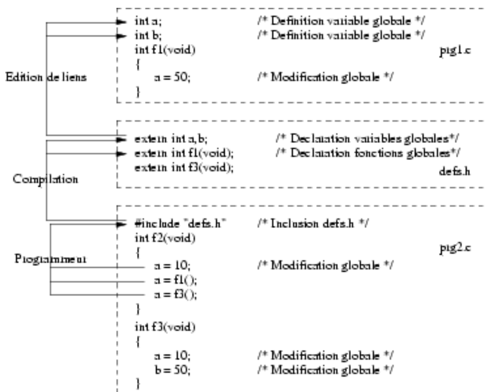
FIG. 9.7 – Utilisation de fichier d'inclusion
