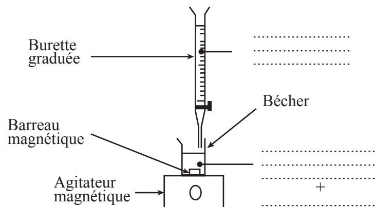
Dispositif d'un dosage colorimétrique
