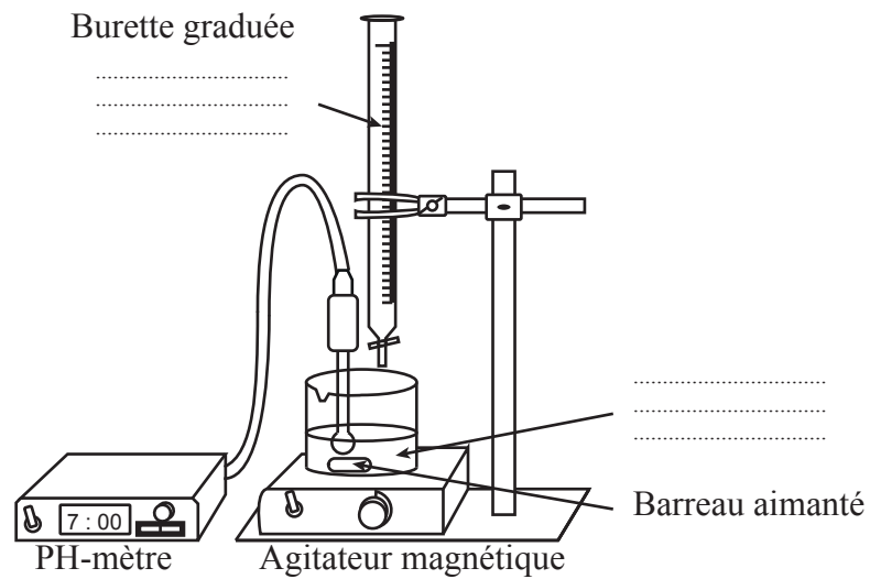
Dispositif d'un dosage pHmétrique
