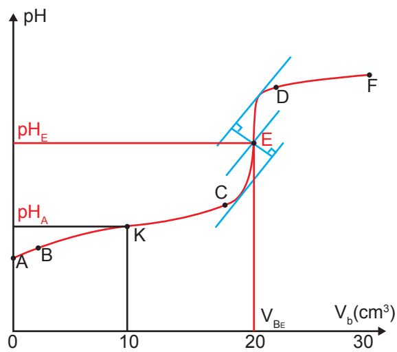
Réaction acide faible - base forte : Courbe de \text{pH} = f(V_b)
