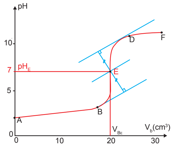
Réaction acide fort - base forte : Courbe de \text{pH} = f(V_b)
