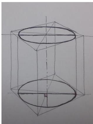
Perspective d'un cercle à deux points de fuite ou vue d'angle
