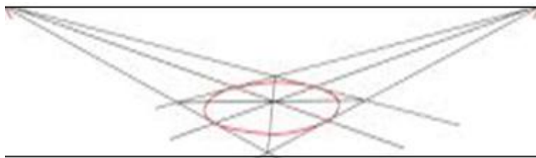
Perspective d'un cercle à deux points de fuite ou vue d'angle
