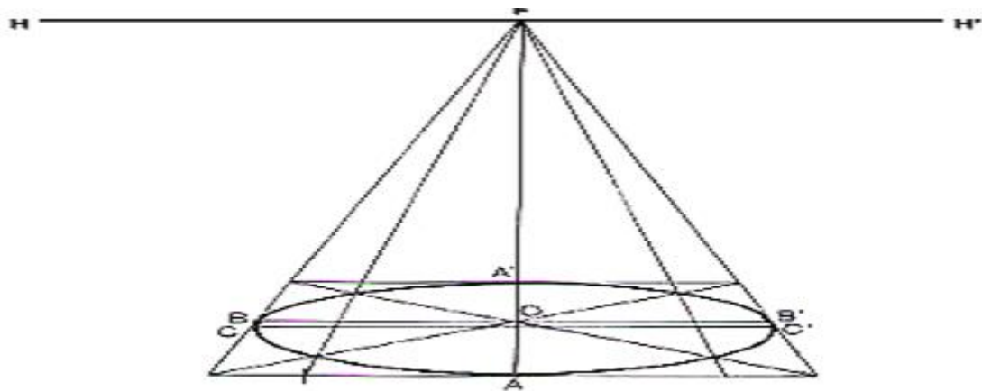
Perspective d'un cercle à un point de fuite ou vue de face
