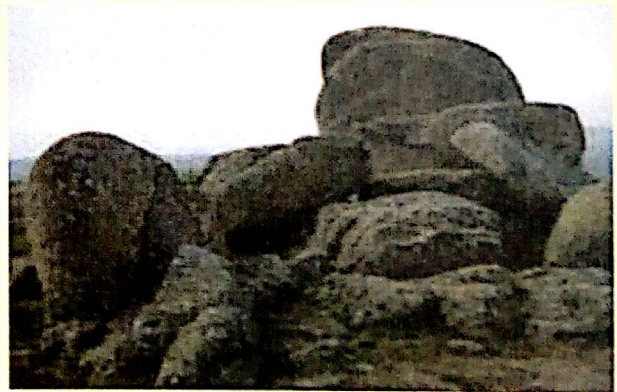
Fig 2 : Un chaos granitique.
