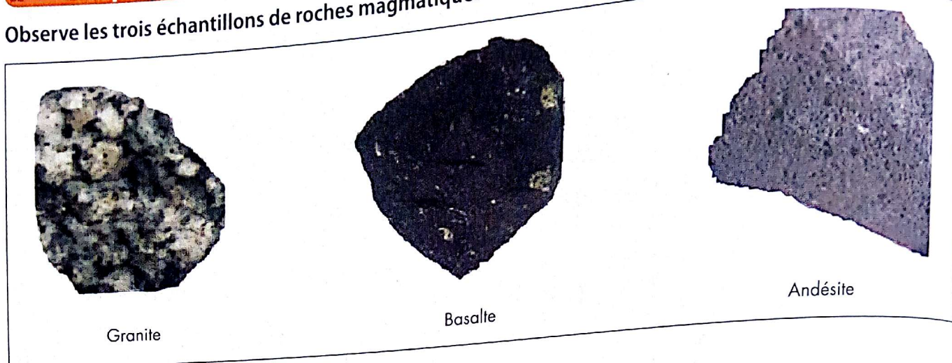
Fig 2 : Trois échantillons de roches magmatiques.
