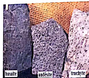
Des roches volcaniques
