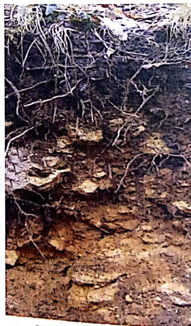
PROFIL D'UN SOL
