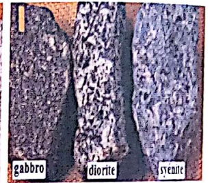
Des roches plutoniques
