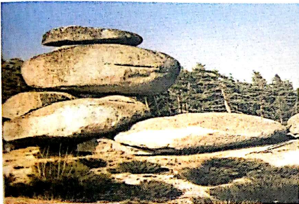
Un chaos granitique.
