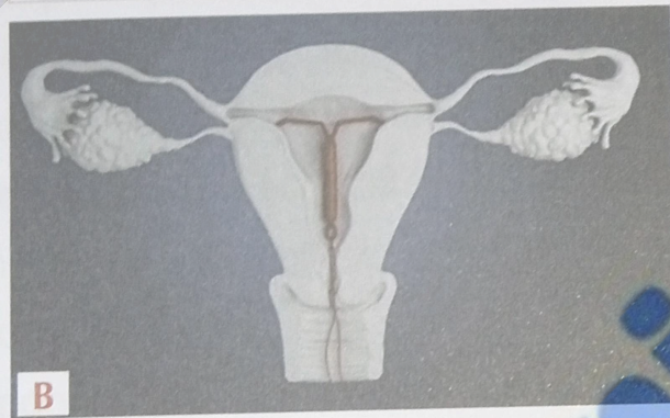
Figure 3 : Le stérilet est un moyen mécanique de lutte contre les grossesses (A et B)
