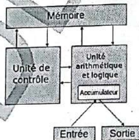
Schématisation de l'architecture de von Neumann.
