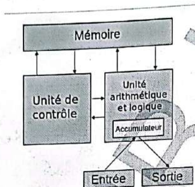
Schématisme de l'architecture de von Neumann.
