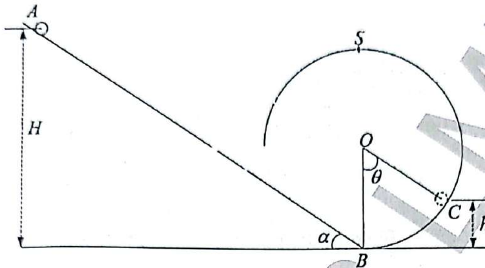
Figure 1: Mouvement d'une particule sur une gouttière
