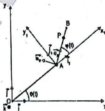
Figure 1: Anneau en mouvement sur une tige.
