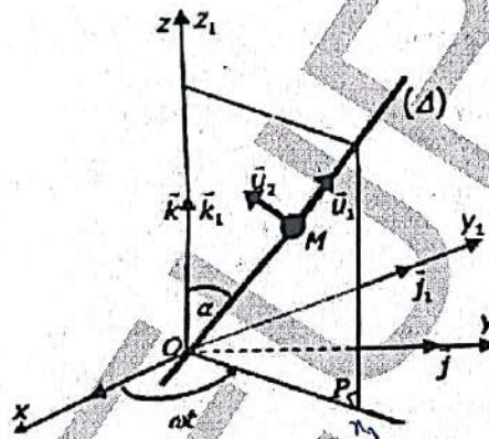
Figure 2: Anneau en mouvement sur une tige.
