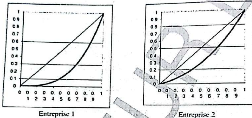
FIGURE 1. Courbes de Lorentz
