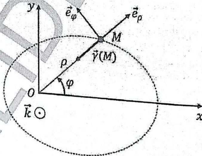
FIGURE 1 – Mouvement à accélération centrale
